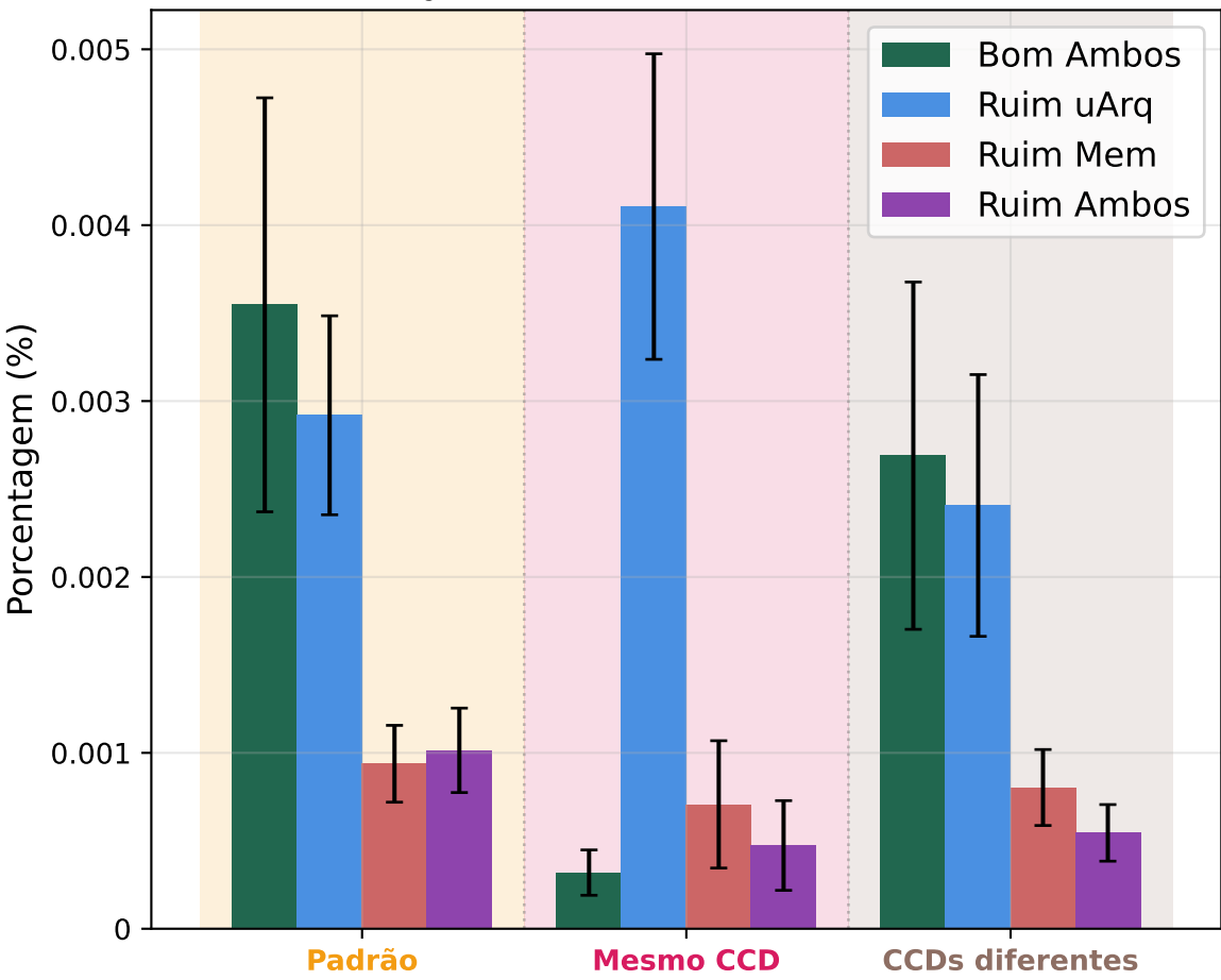
Contenção SMT (% de Ciclos) (3 Threads)
