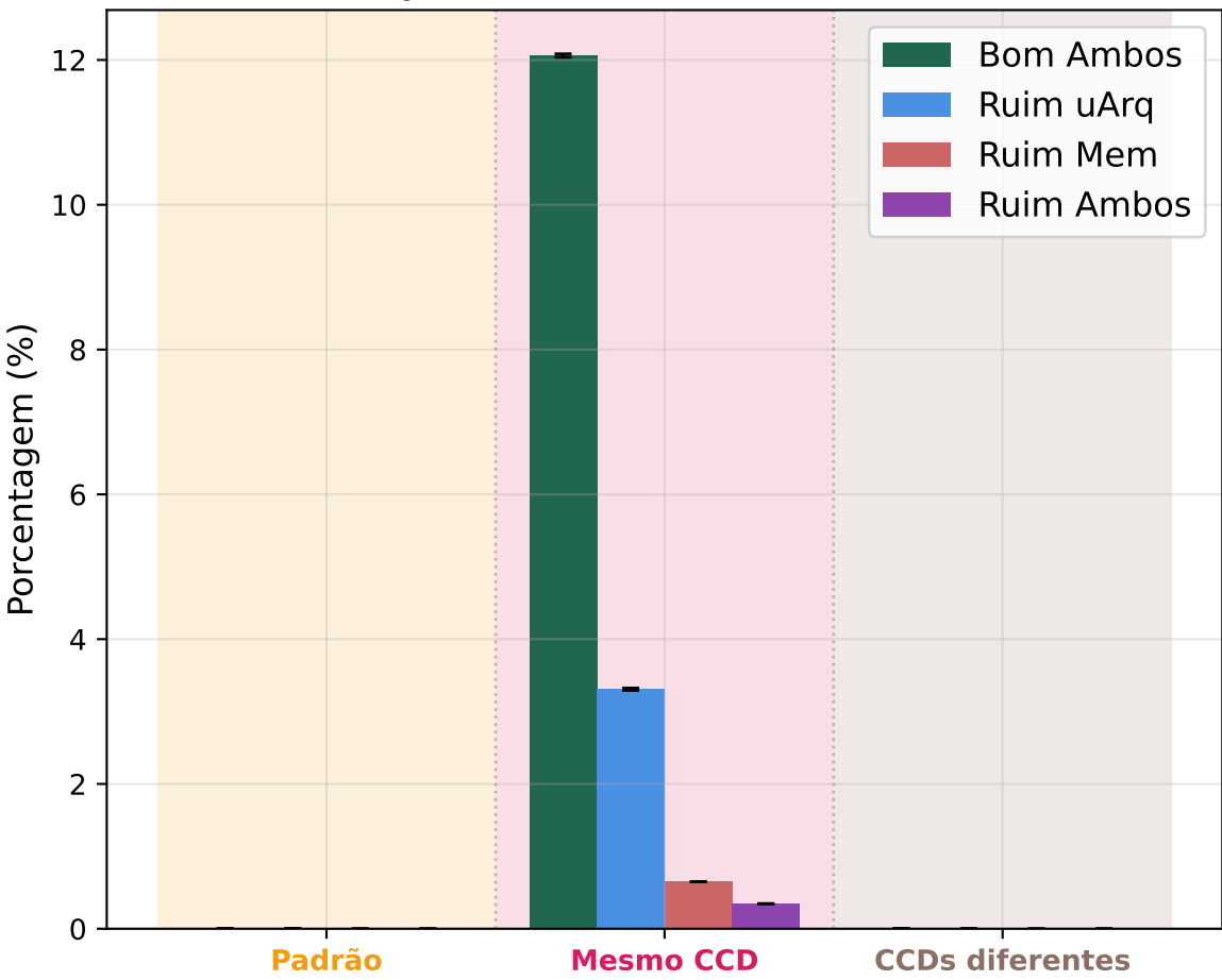
Contenção SMT (% de Ciclos) (7 Threads)
