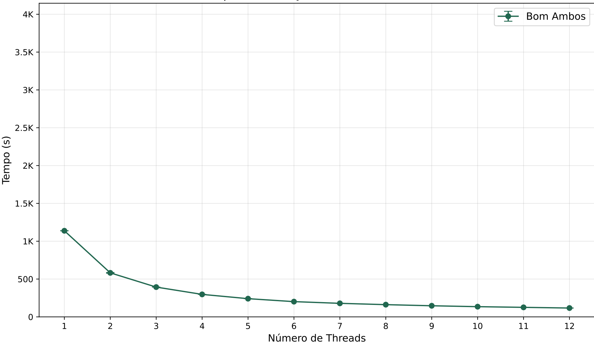
Tempo de Execução vs Threads (Padrão)
