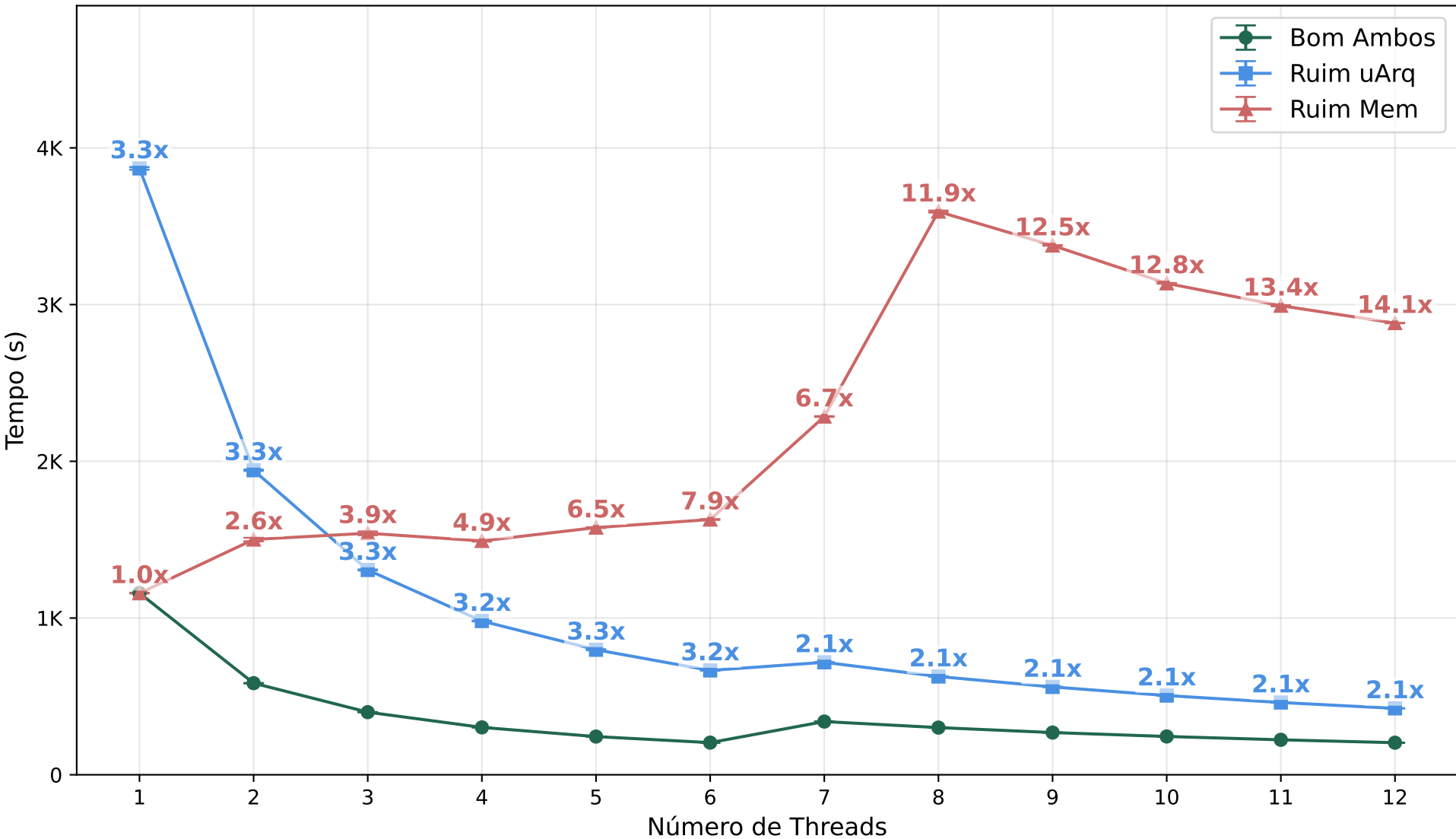
Tempo de Execução vs Threads (Mesmo CCD)
