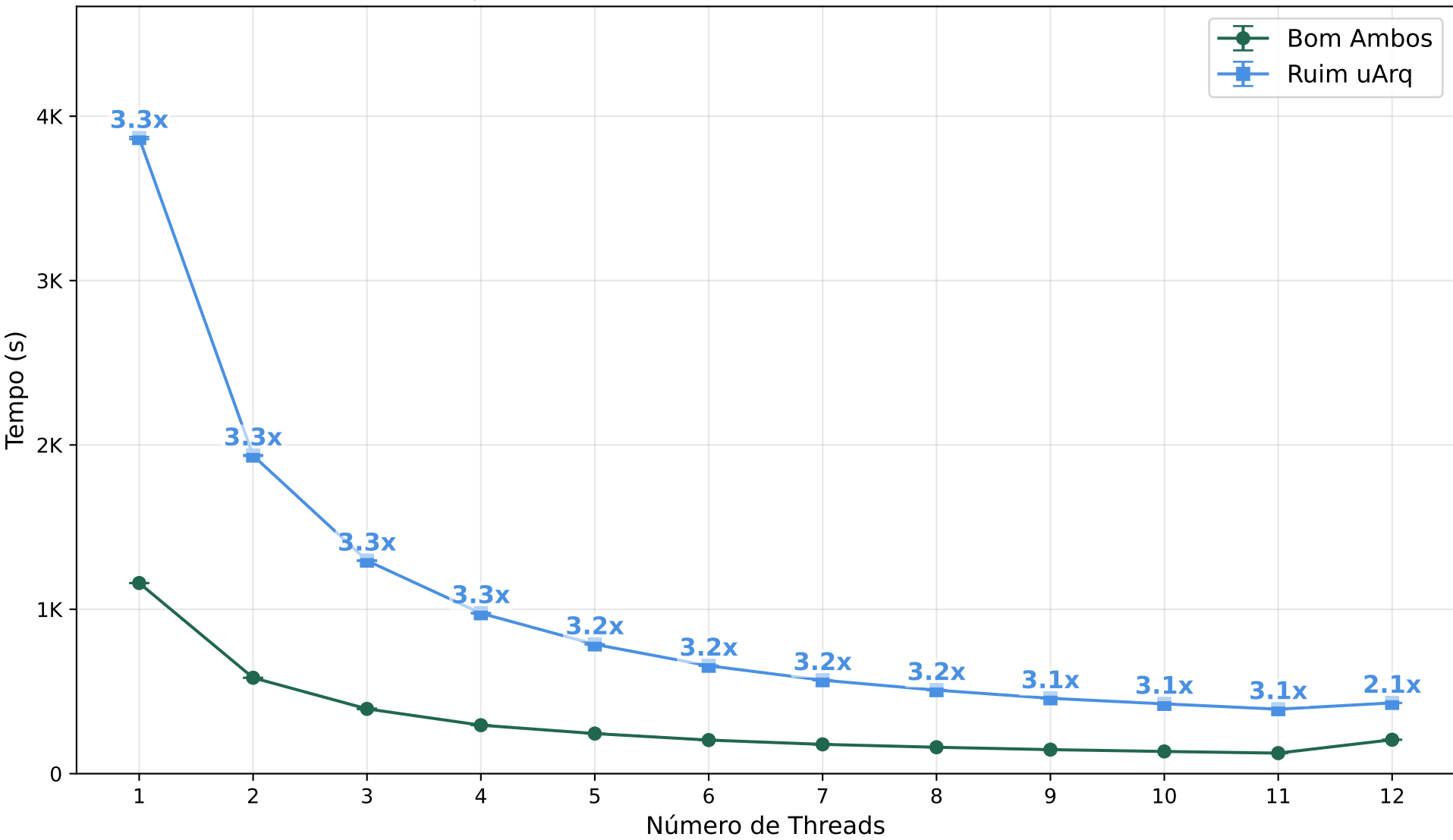
Tempo de Execução vs Threads (CCDs diferentes)
