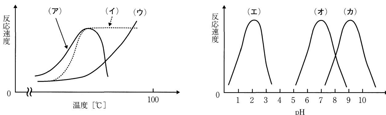
図3 温度、pHと反応速度の関係
