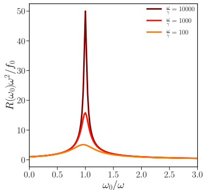
図 5: 振動振幅 R(\omega_0) の外力の振動数 \omega_0 依存性. 不足減衰条件の様子を図示したもの. \omega/\gamma が大きいとき \omega_0 \sim \omega で R(\omega_0) はピークを示す. ただし厳密には, ピーク位置は \omega_0^* = \sqrt{\omega^2 - 2\gamma^2} = \omega\sqrt{1 - 2(\gamma/\omega)^2} . \omega/\gamma の減少にともないピークが低振動数側にシフトし, その高さは低くなる.
