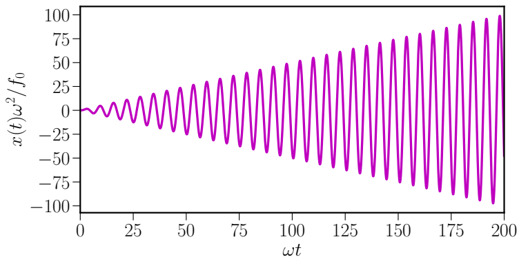
図 4: \omega_0/\omega = 1 : 共鳴時における特殊解 (23) の振る舞い.
