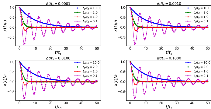
図 1: 数値計算結果。パラメータ \zeta^* = \frac{t_s}{t_d} を変化した時の様子。 \zeta^* = 2 が臨界減衰であり、これを境に振る舞いが大きく変化している様子が見てとれる。また数値計算の収束性をいくつかの \Delta t で確認。 \Delta t = 0.1 でもそれなりに計算ができていている様子が見てとれる。ただし誤差は O(\Delta t) で生じている。
