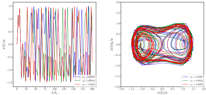
図 5: f^* = 0.40 における x(t) の t 依存性および位相図.
