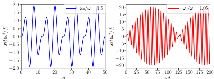
図 3: 強制振動の特殊解：式 (23) の時間依存性. (左) \omega_0/\omega = 1.5 の時. (右) \omega_0/\omega = 1.05 の時. \omega と \omega_0 が近い時は, うなりの様子が見て取れる. ここでの短周期振動の周期 T_1 は \omega T_1 = 4\pi\omega/(\omega_0 + \omega) \sim 6.1 , 長周期振動の周期 T_2 は, \omega T_2 = 2\pi\omega/(\omega_0 - \omega) = 40\pi \sim 125 となる.
