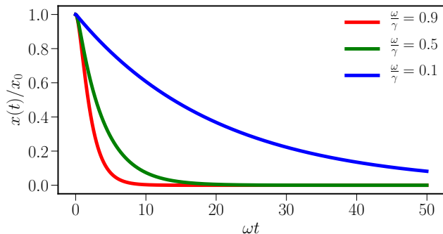
図 3: パラメータを変化させた式 (34) の曲線を図示したもの．減衰の様子が見て取れる．パラメータ \omega/\gamma が 1 より小さくなるほど、緩和が遅くなる． \omega/\gamma \rightarrow 0 極限ではほとんど減衰なくなり停止しているように振舞う．
