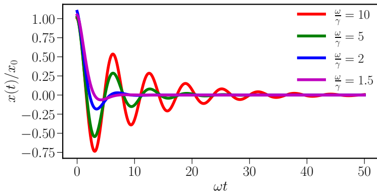
図 2: 式 (26) をパラメータを変化させ図示したものであり、減衰振動の様子が見て取れる。式 (26) は、 x(t)/x_0 = \frac{1}{\sqrt{1-(\gamma/\omega)^2}} e^{-(\gamma/\omega)\omega t} \sin(\sqrt{1-(\gamma/\omega)^2}\omega t + \phi) , \tan \phi = \sqrt{(\omega/\gamma)^2 - 1} と表されるので、グラフの軸の横軸を \omega t (無次元数)、縦軸を x(t)/x_0 (無次元数) とすれば、曲線は \omega/\gamma をパラメータとして一意に定まる。パラメータ \omega/\gamma が 1 に近づくほど、振動が弱くなる。( \omega/\gamma = 1 を臨界減衰条件といい、後で扱う。 )
