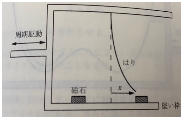
図 1: Duffing 振動子の実験例：磁気弾性力力学系（ストロガッツ著：非線形ダイナミクスとカオス（丸善）より抜粋）。
