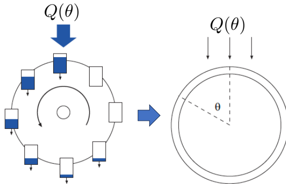
図 2: カオス水車の模式図. 左: 有限個のコップを取り付けた水車. 右: 無限個のコップからなる水車 (連続体極限). 守田智「ローレンツ水車によるカオスの実演とその数理」より引用. 動画:
