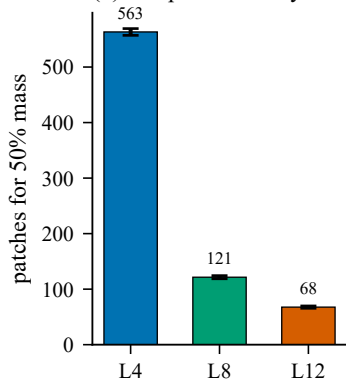
(d) L4 spreads widely
