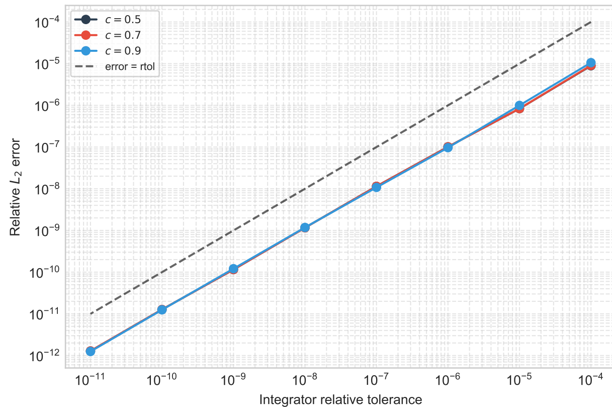
Classical diffusion
