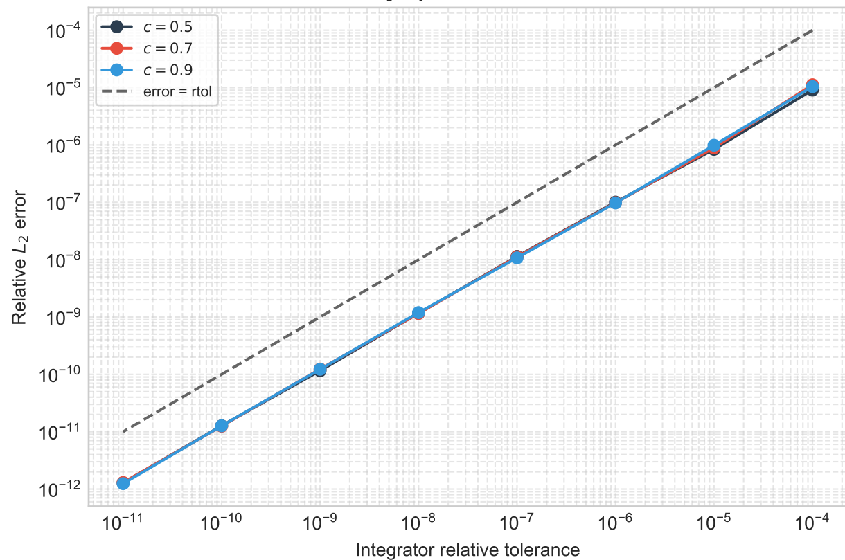
Asymptotic diffusion
