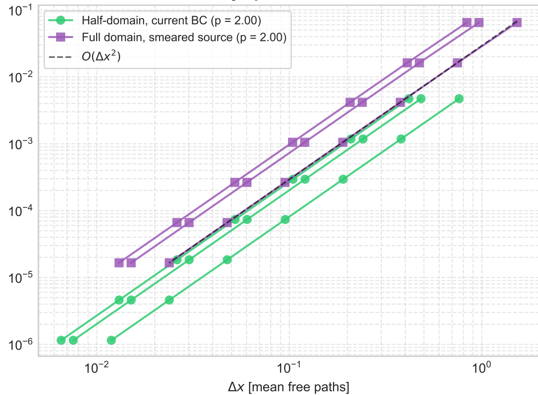
Asymptotic diffusion
