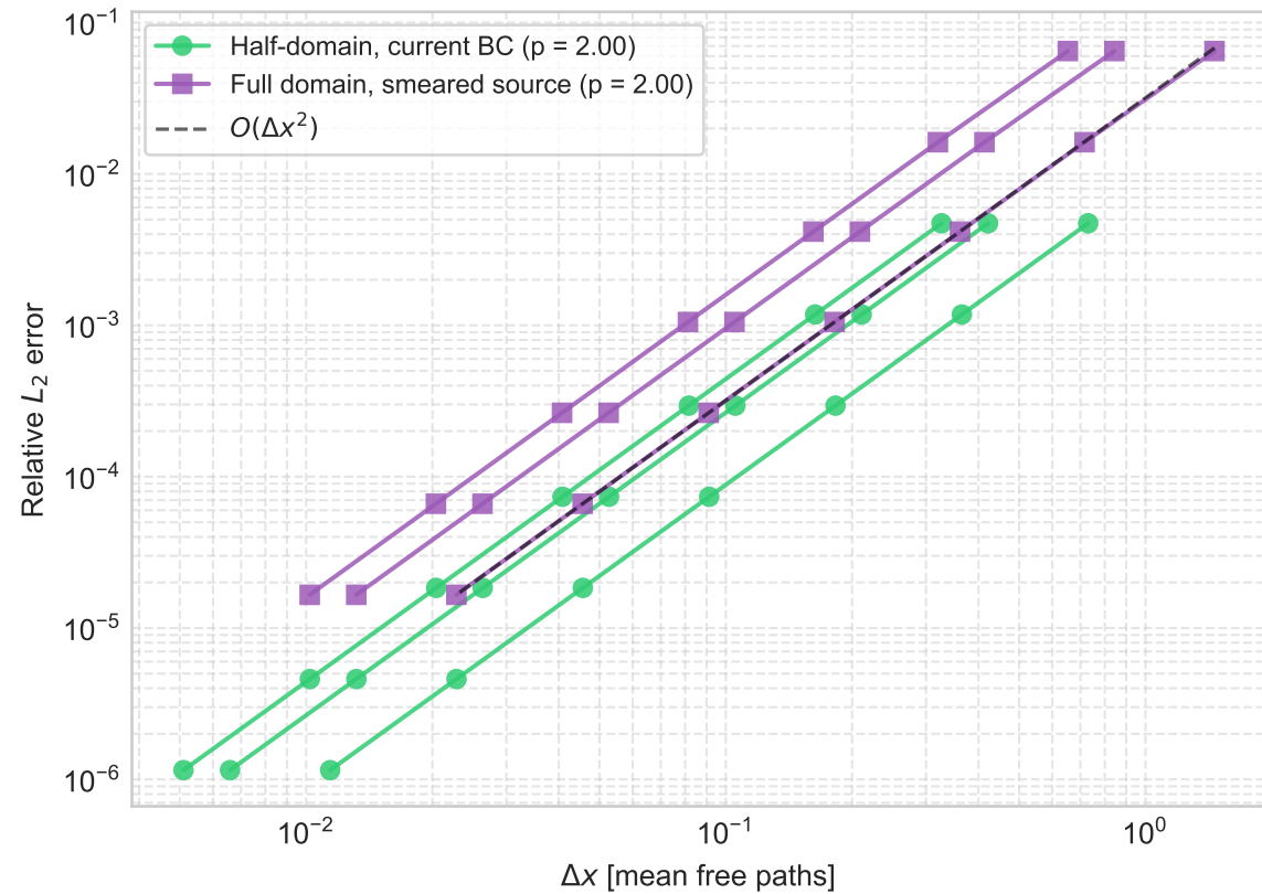
Classical diffusion
