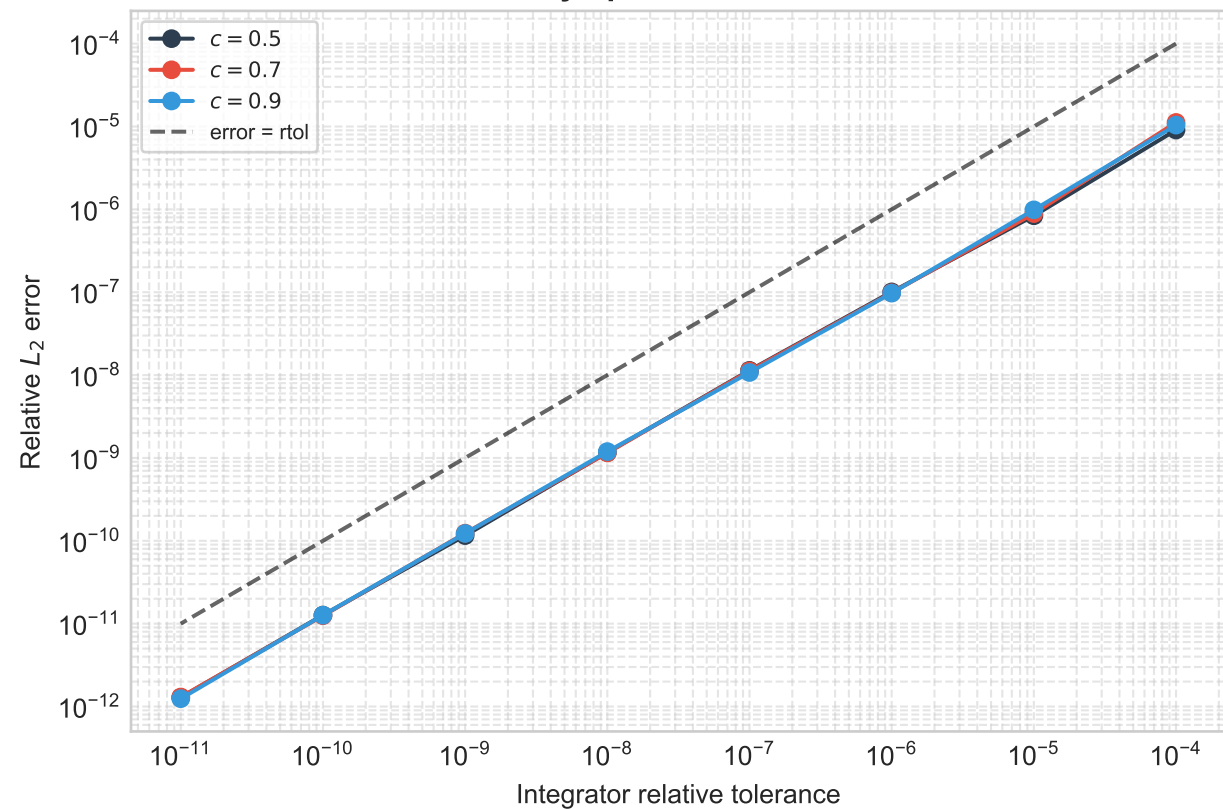
Asymptotic diffusion
