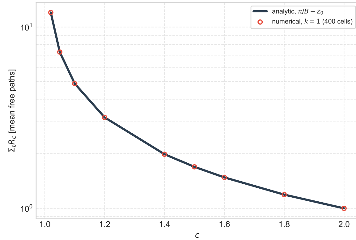
Asymptotic diffusion
