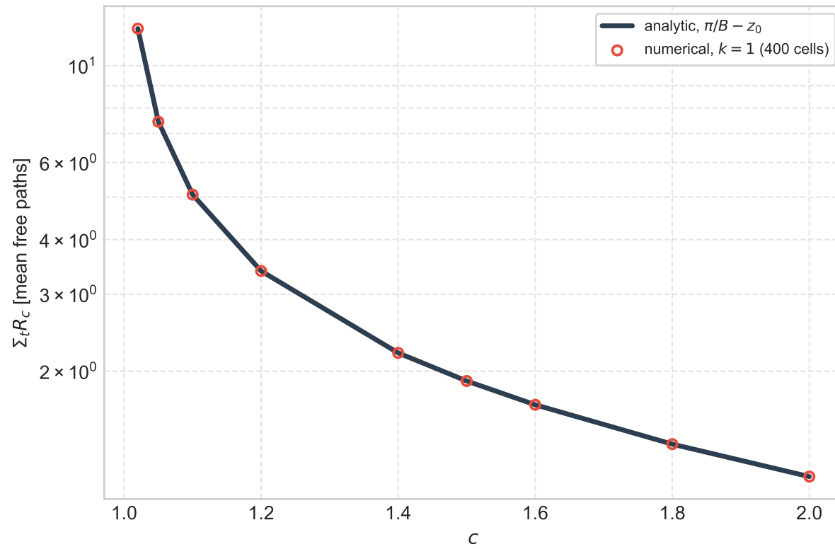
Classical diffusion
