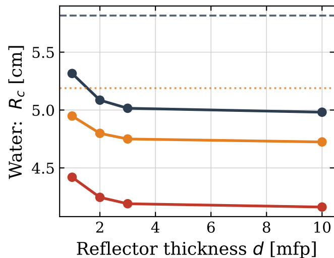
Pu-239
