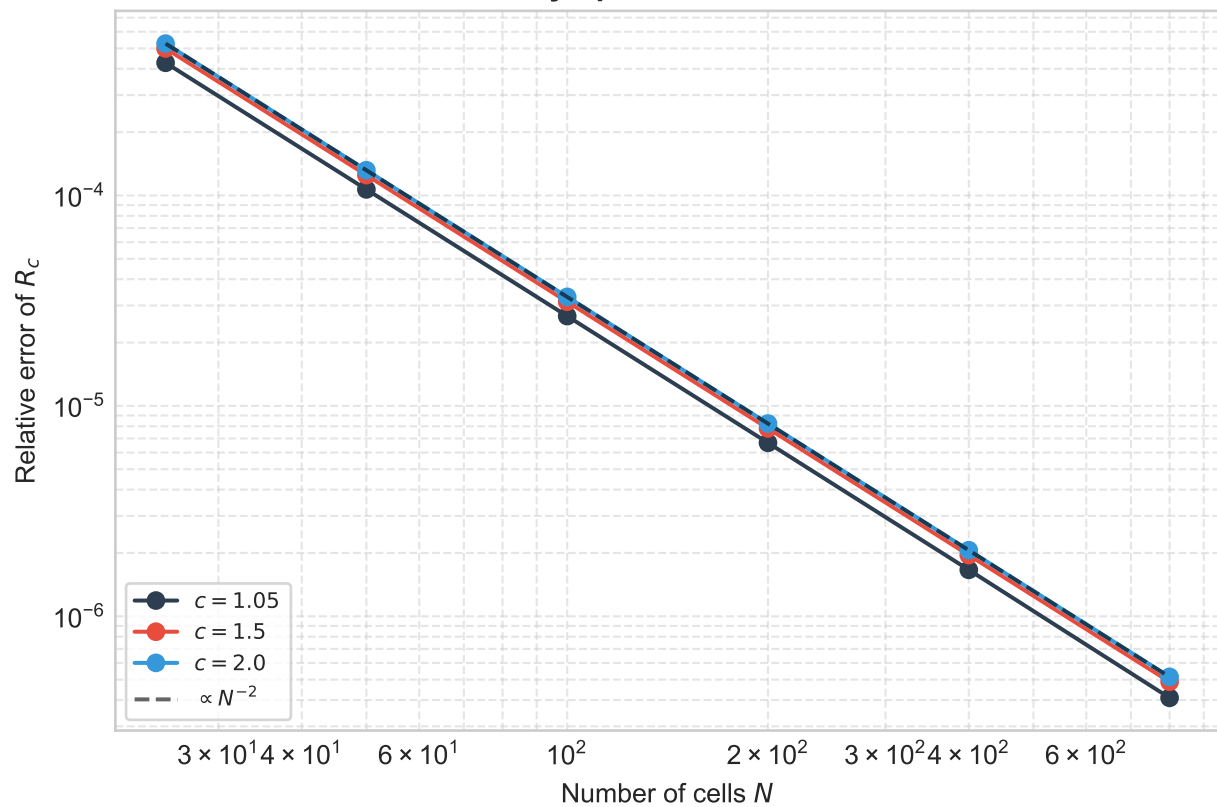
Asymptotic diffusion
