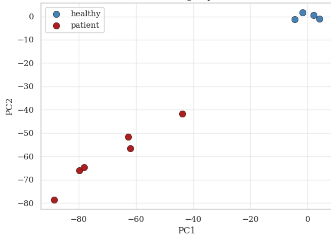
PCA — true group labels
