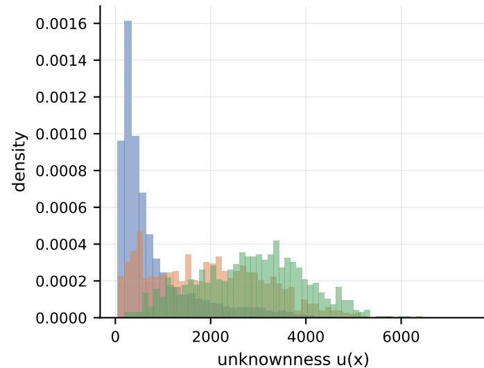
MAHALANOBIS
