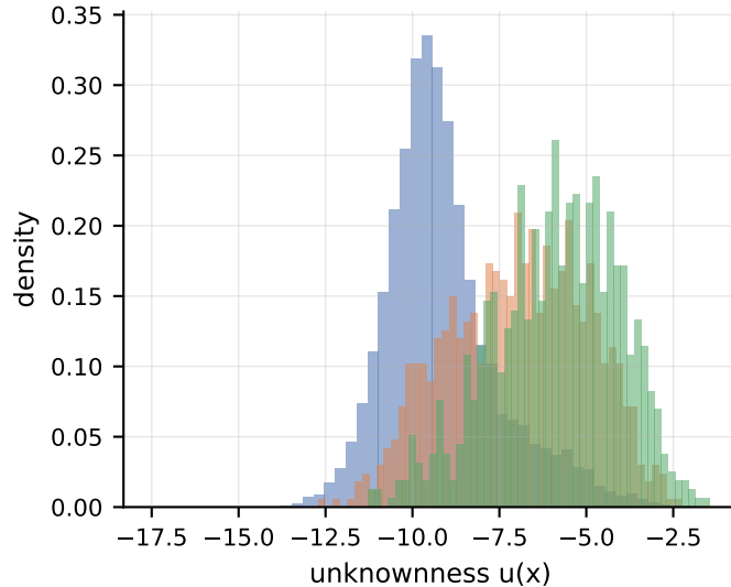
MLS
