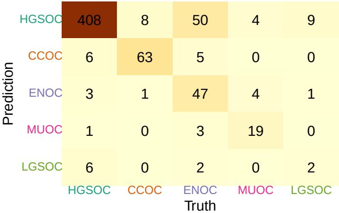
Up-XGB
