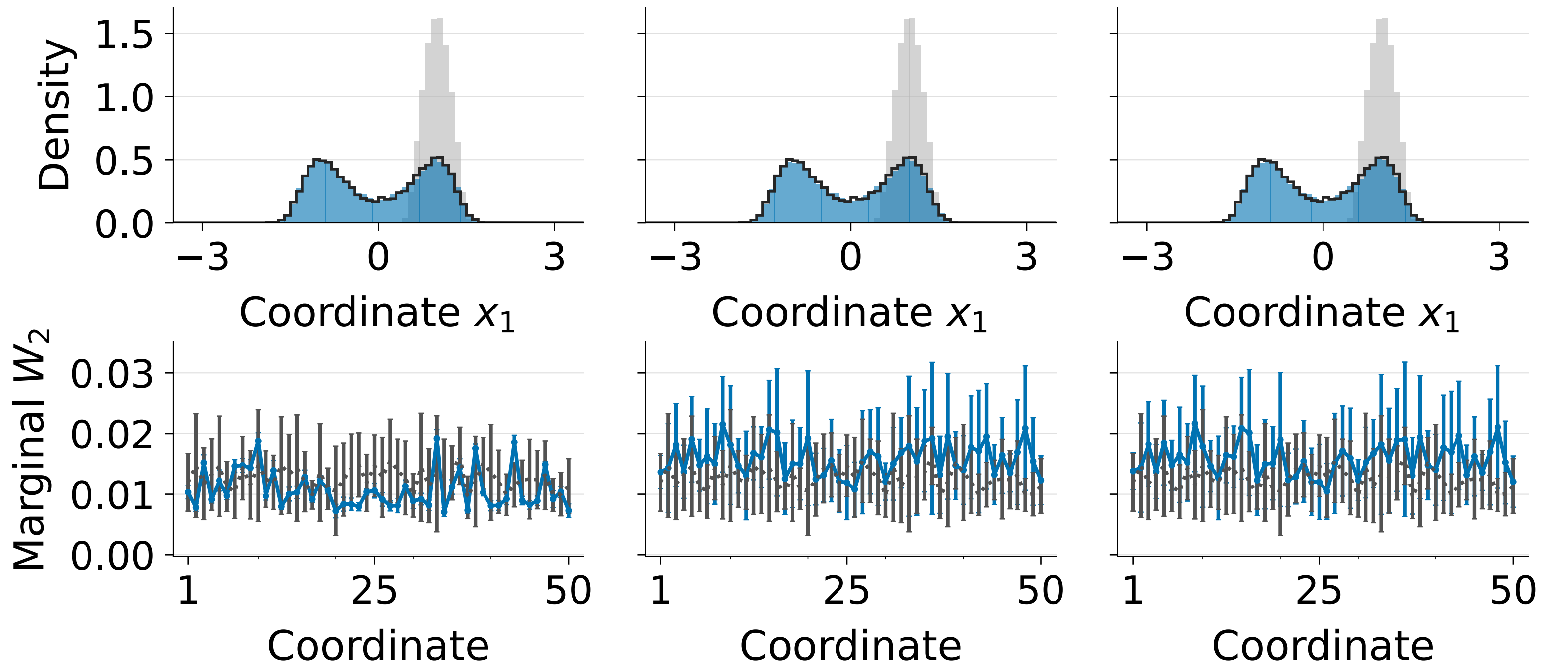
Koopman (RBF)
