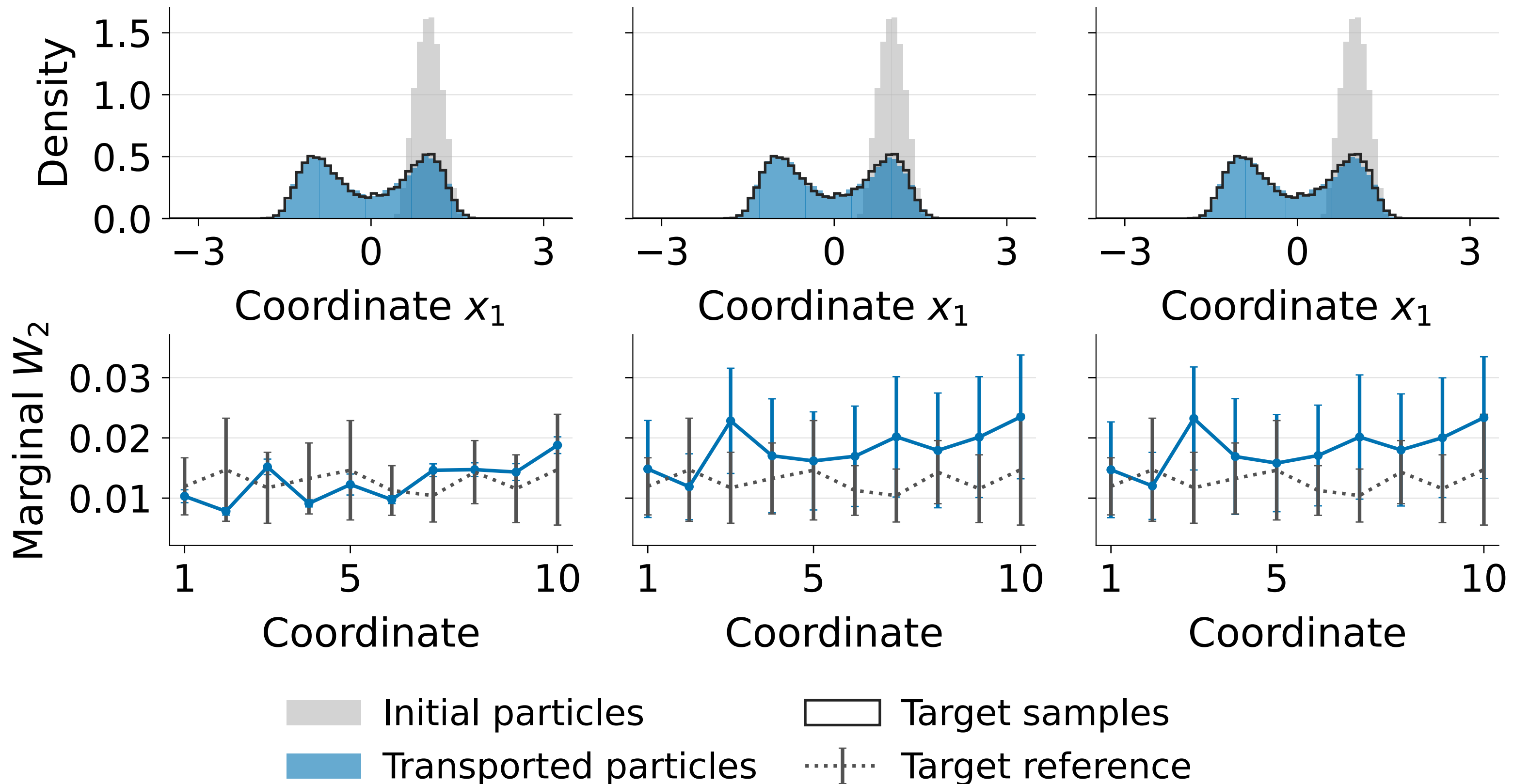
Koopman (RBF)
