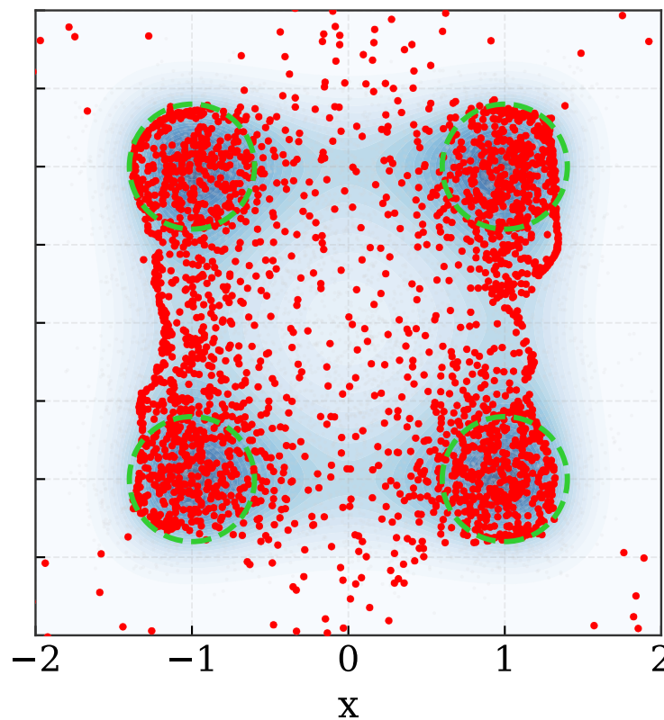
KSWGd: step 1000
