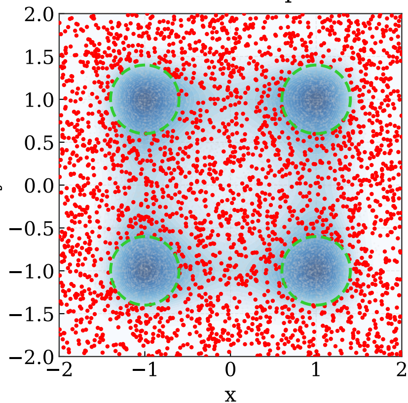
KSWGd: step 0
