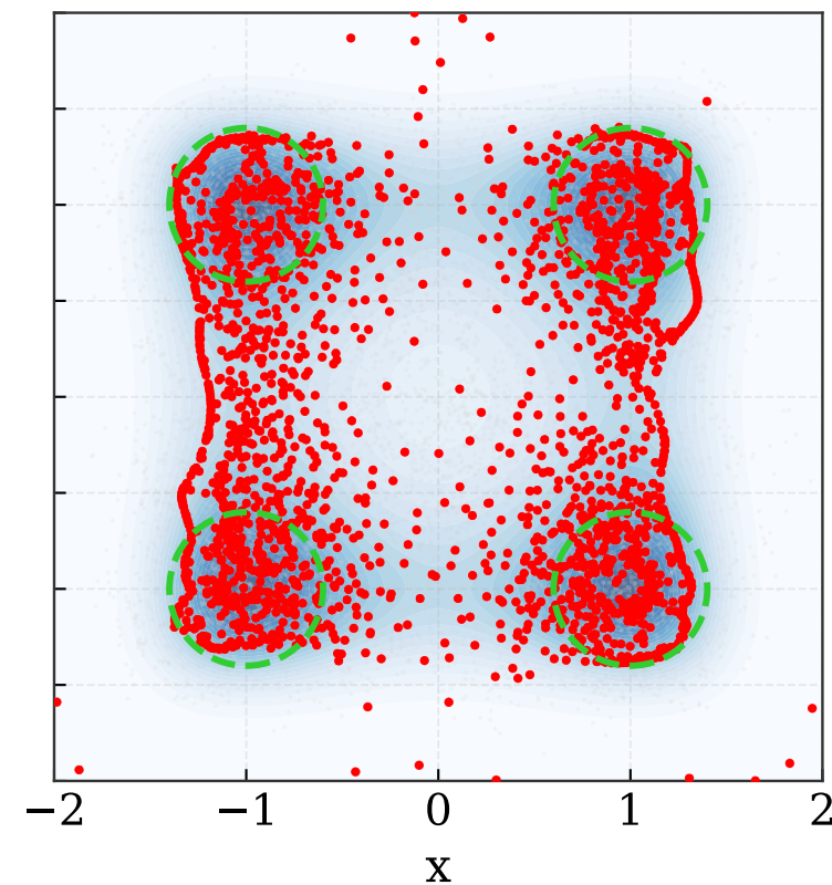
KSWGd: step 3000
