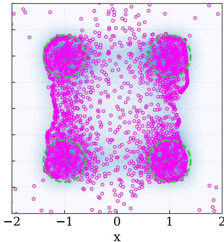
KSWGd: step 1000
