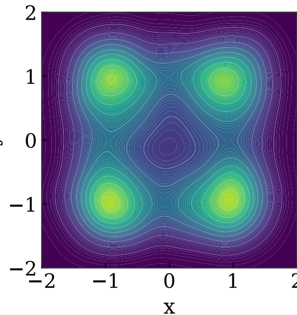
ULA
