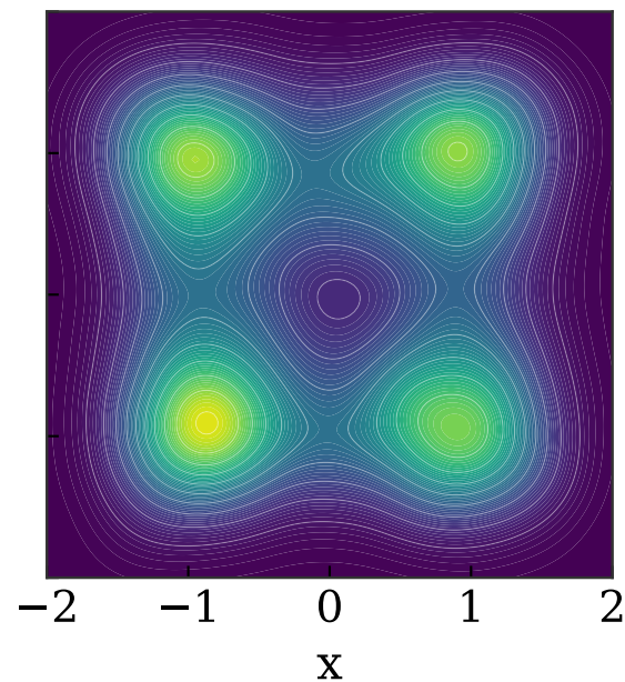
MALA
