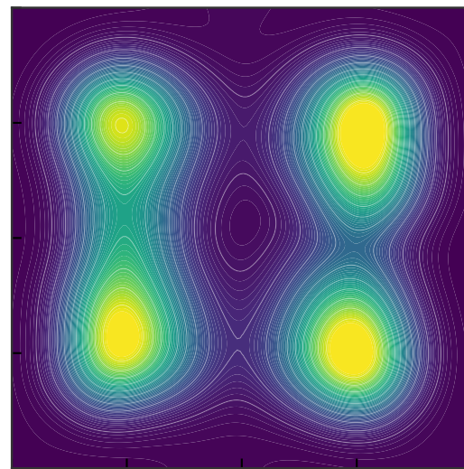
KSWG
