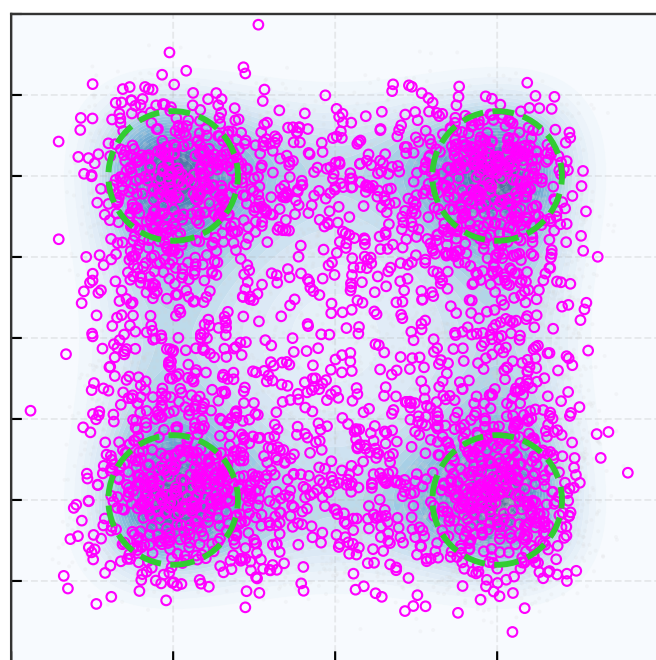
MALA: step 1000
