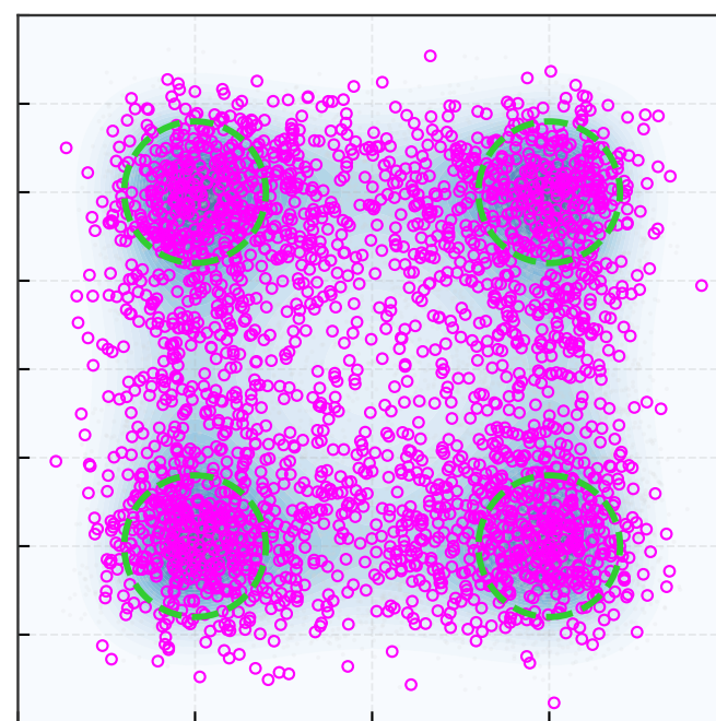
MALA: step 3000
