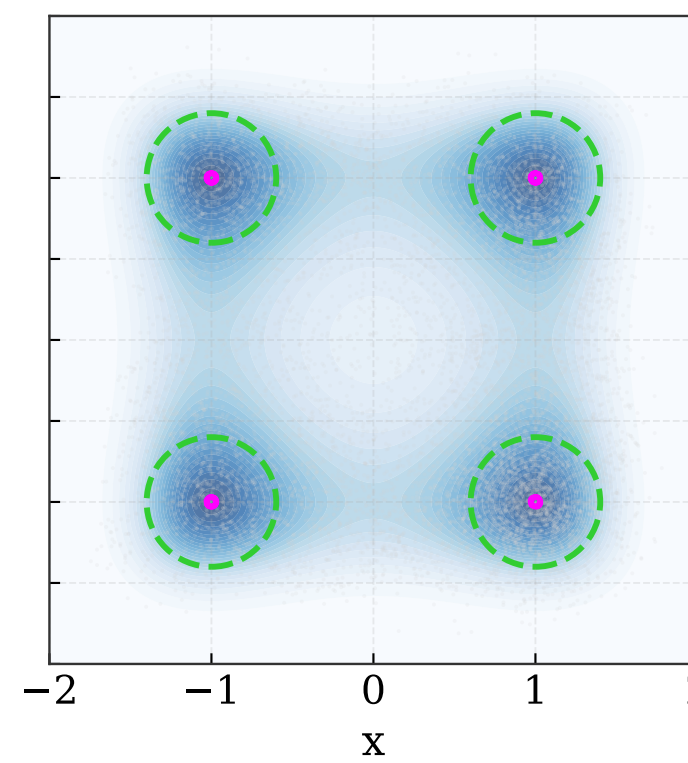
LDVI: step 3000
