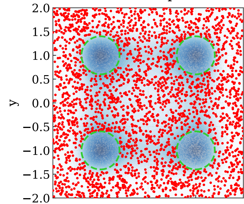
MALA: step 0
