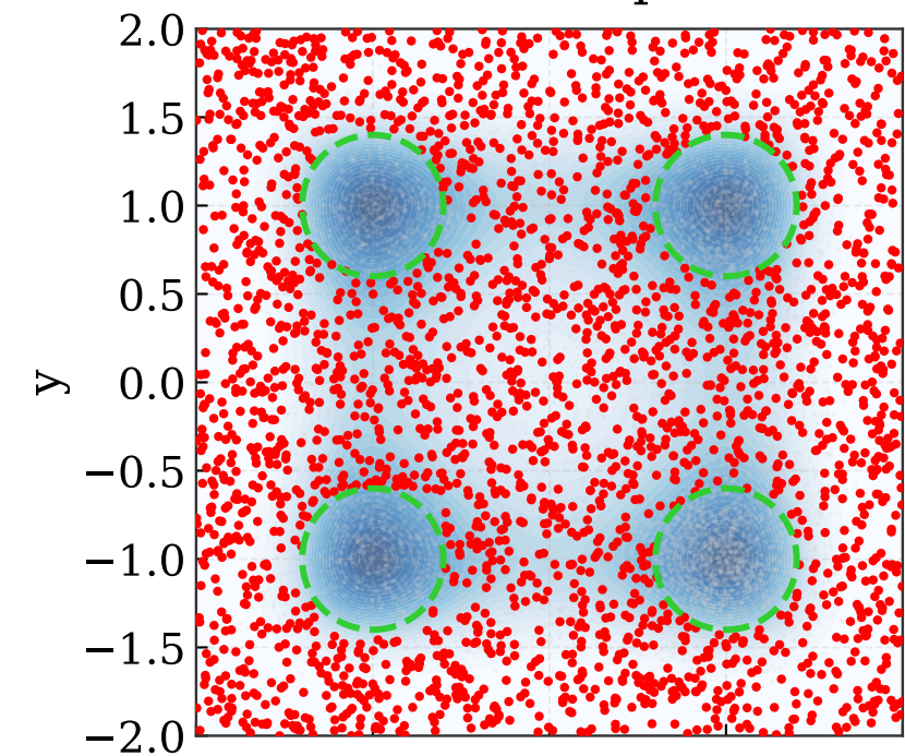
LDVI: step 0
