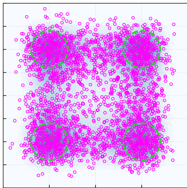
ULA: step 1000
