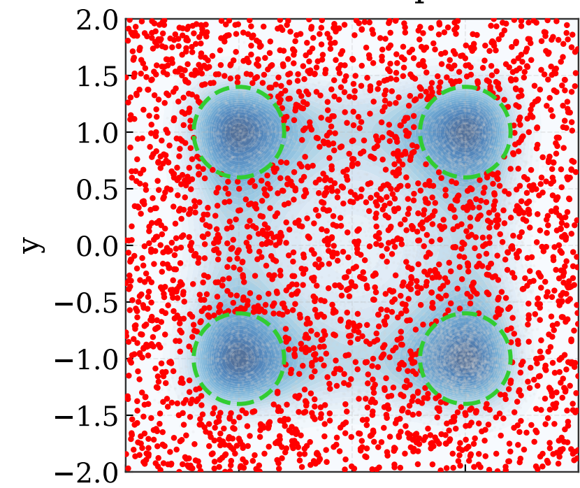
ULA: step 0
