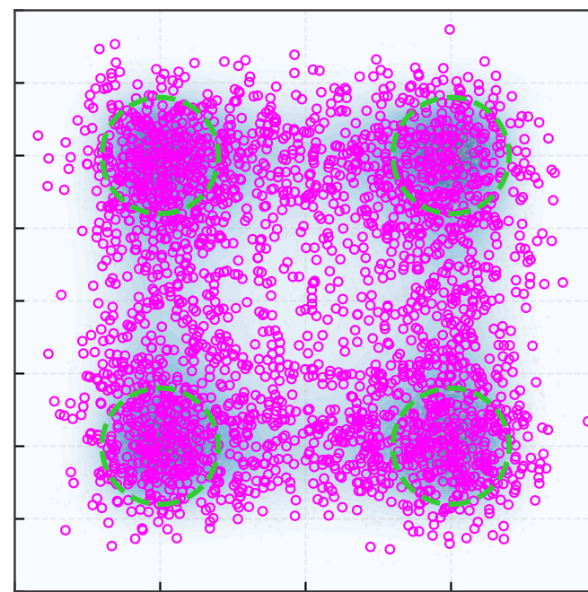
ULA: step 3000
