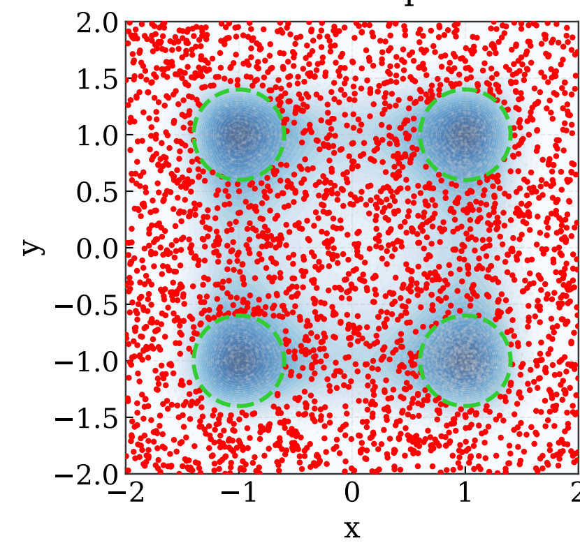
LDVI: step 0
