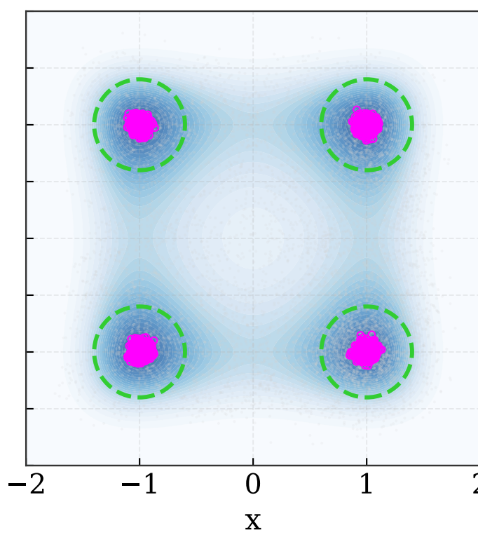
LDVI: step 1000
