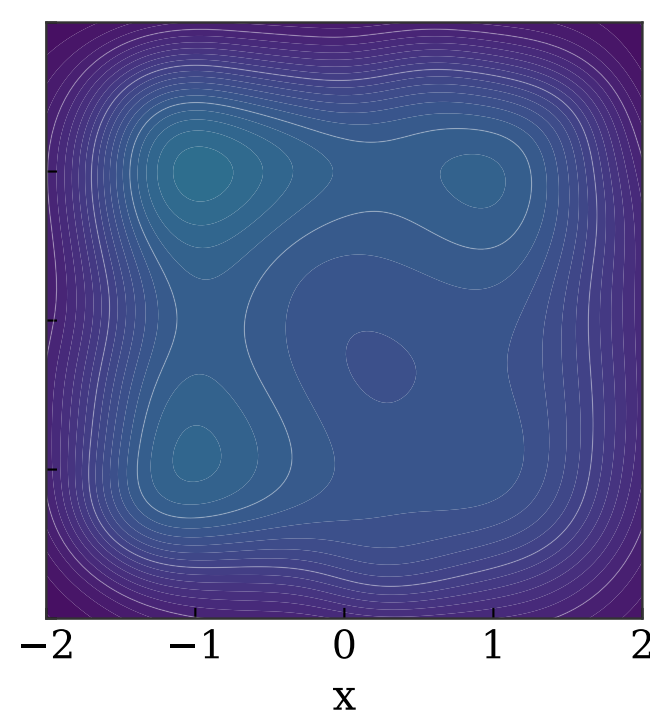
DMPS (Step 3000)
