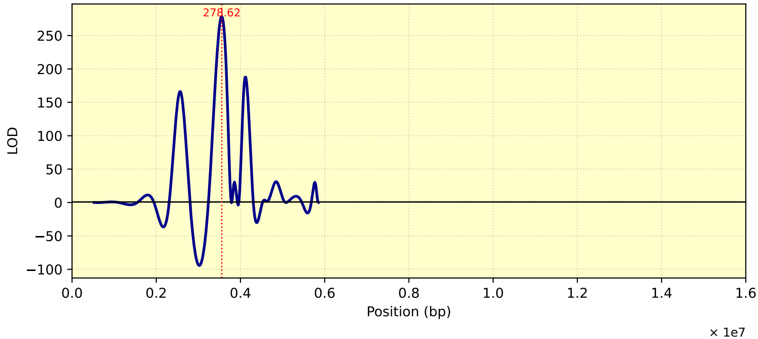
LOD Curve - chr18 - Tc27triKT
