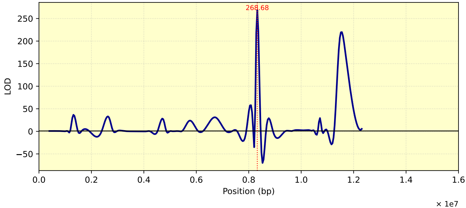
LOD Curve - chr02 - Tc27triKT
