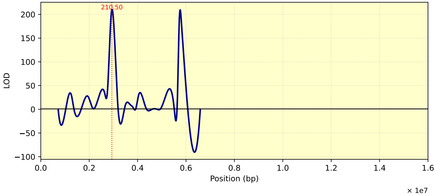
LOD Curve - chr13 - Tc27triKT
