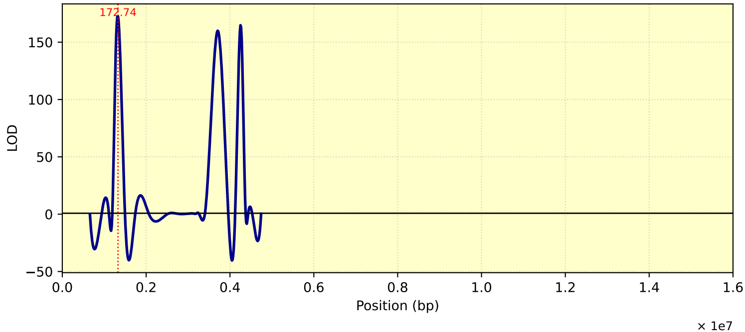
LOD Curve - chr21 - Tc27triKT
