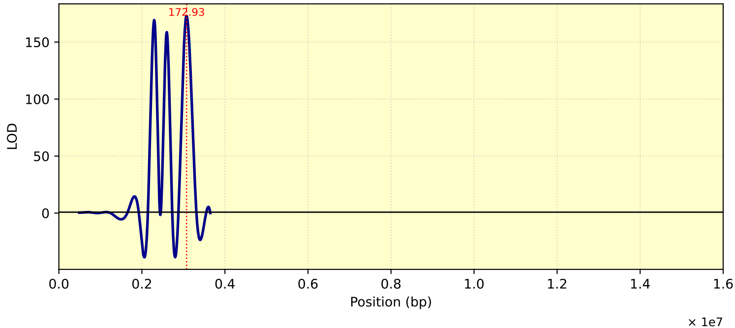
LOD Curve - chr24 - Tc27triKT
