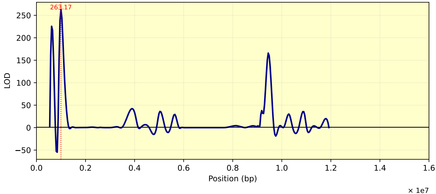
LOD Curve - chr05 - Tc27triKT
