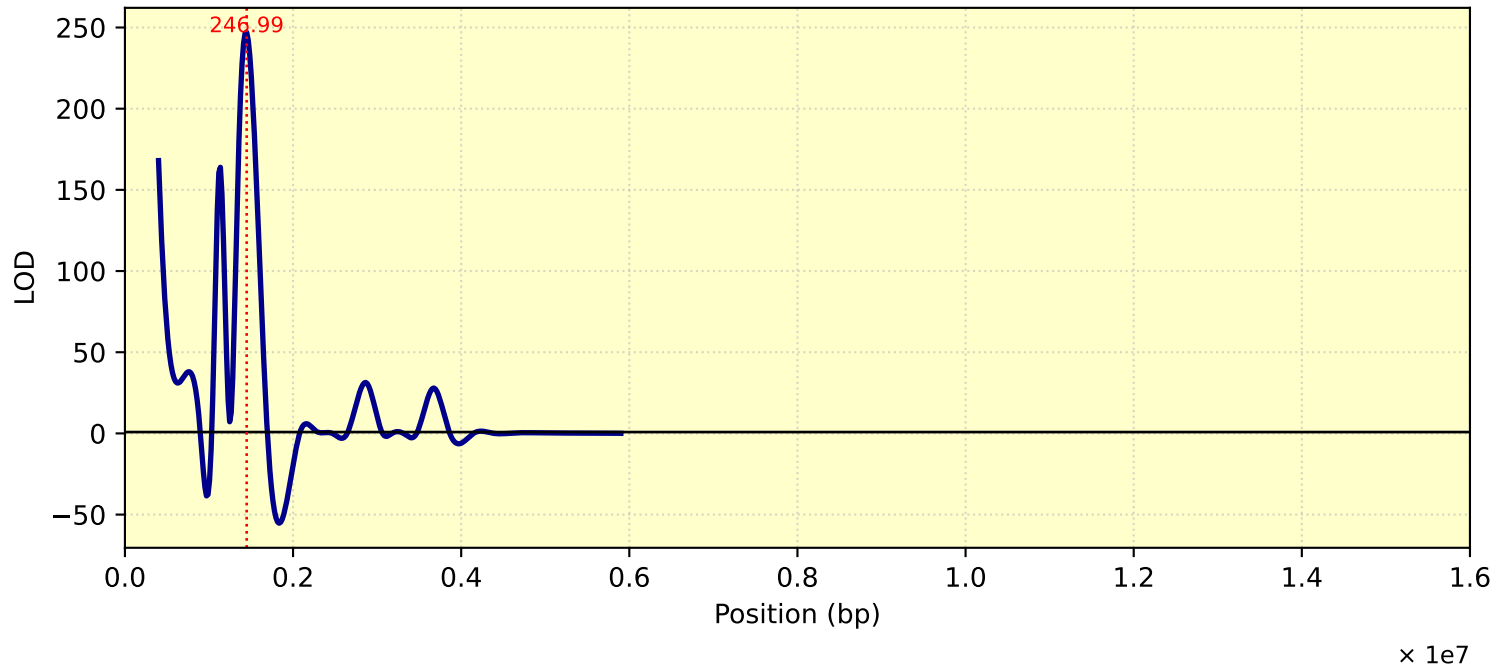
LOD Curve - chr14 - Tc27triKT
