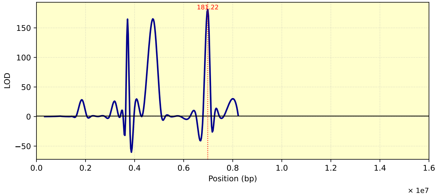
LOD Curve - chr07 - Tc27triKT
