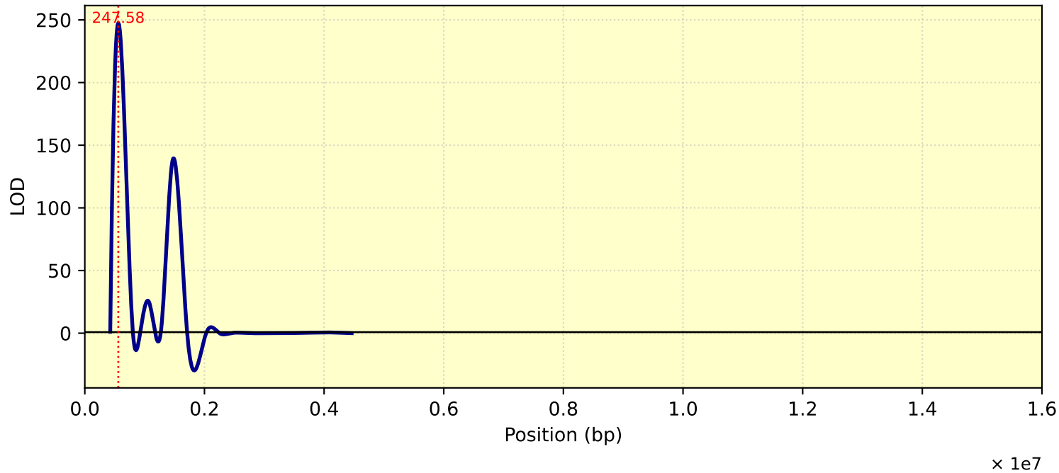
LOD Curve - chr22 - Tc27triKT
