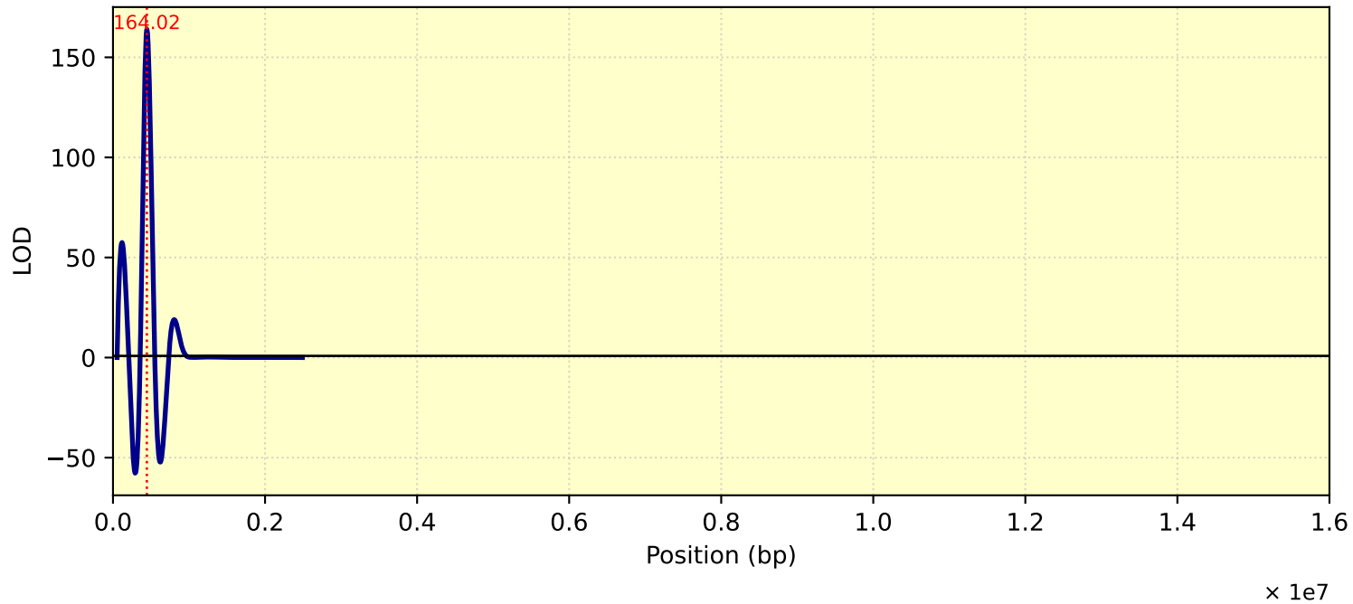
LOD Curve - chr25 - Tc27triKT
