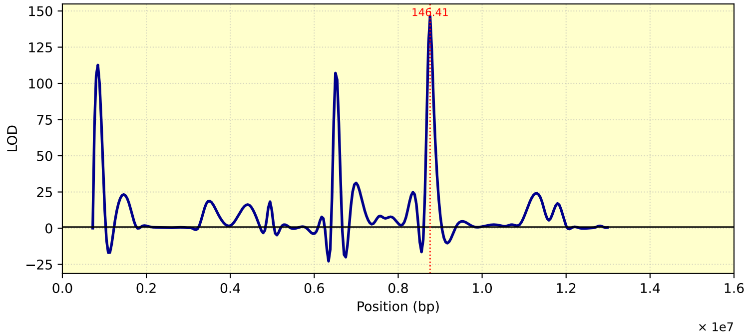
LOD Curve - chr09 - Tc30me2
