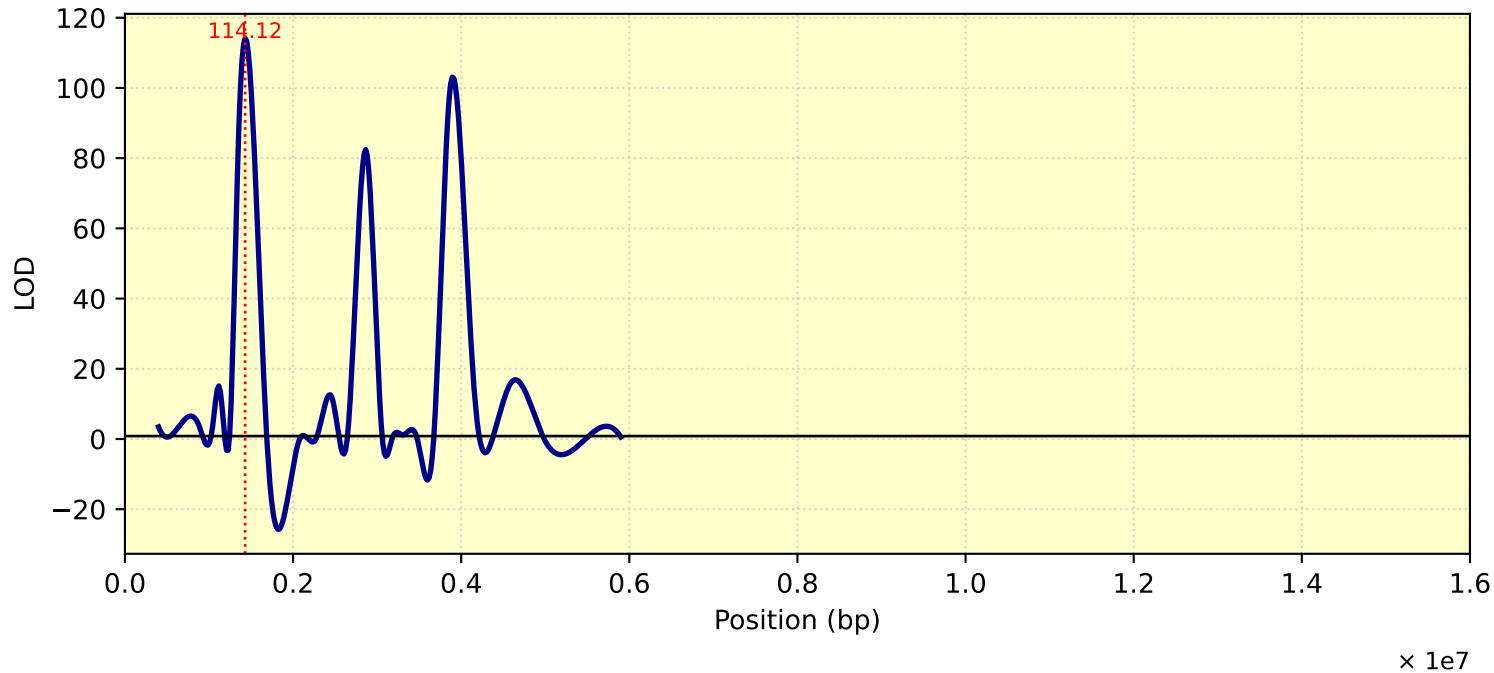
LOD Curve - chr14 - Tc30me2
