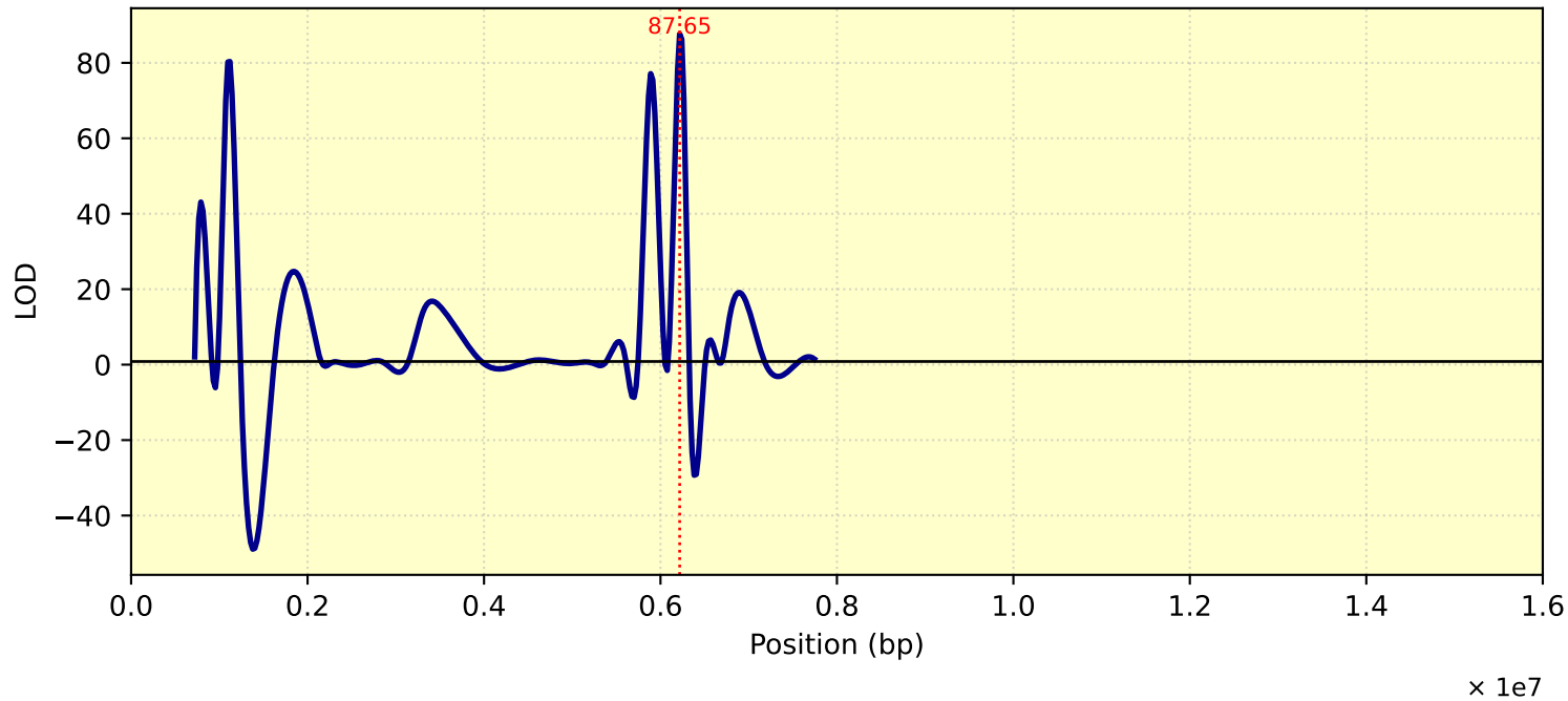
LOD Curve - chr08 - Tc30me2
