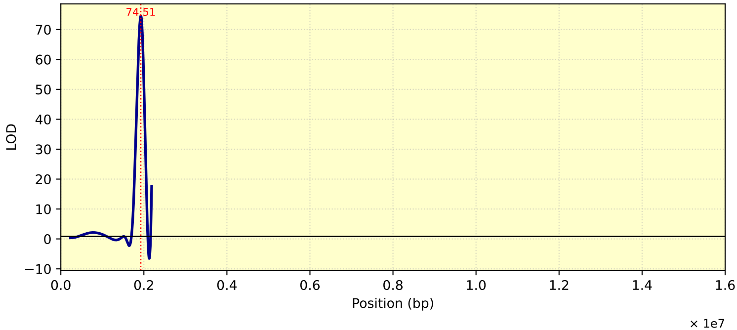
LOD Curve - chr23 - Tc30me2
