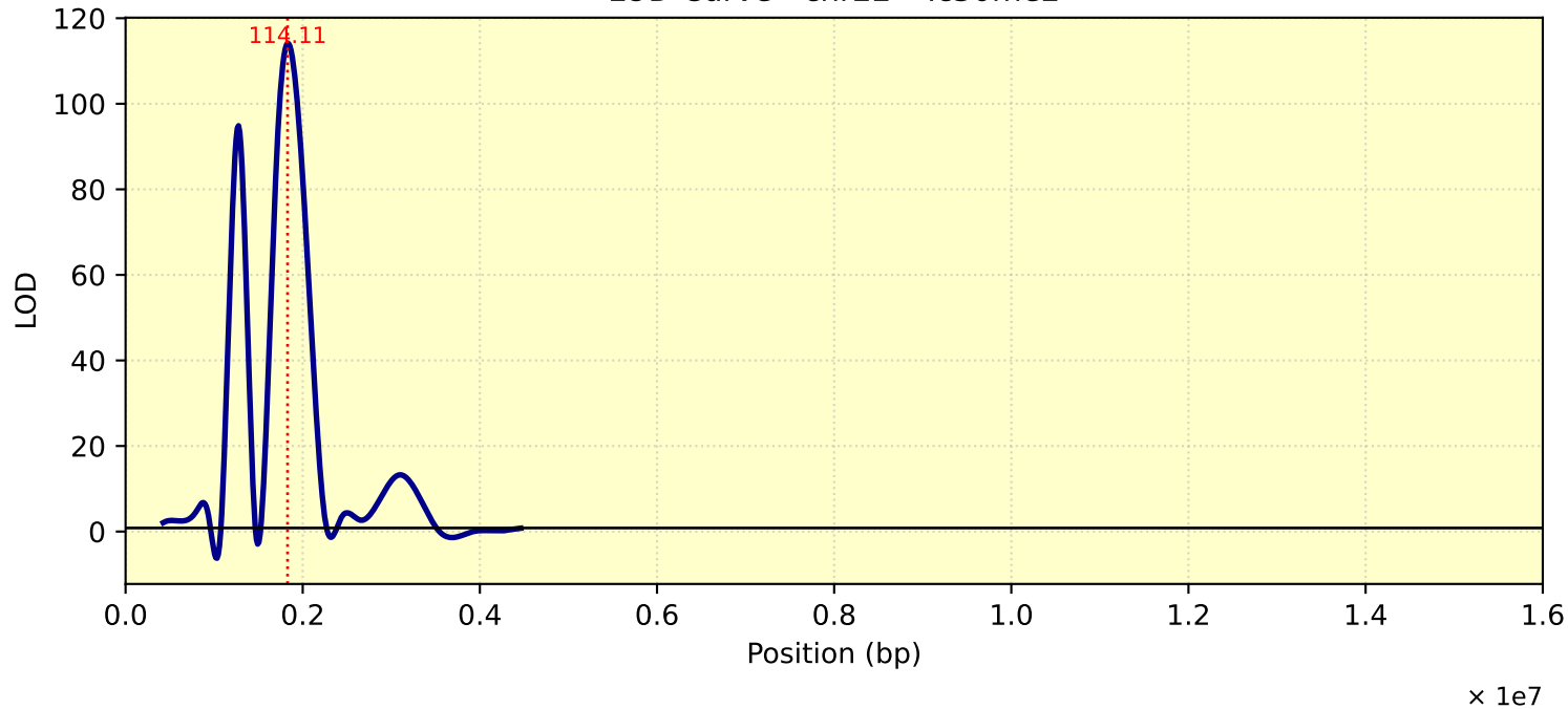
LOD Curve - chr22 - Tc30me2
