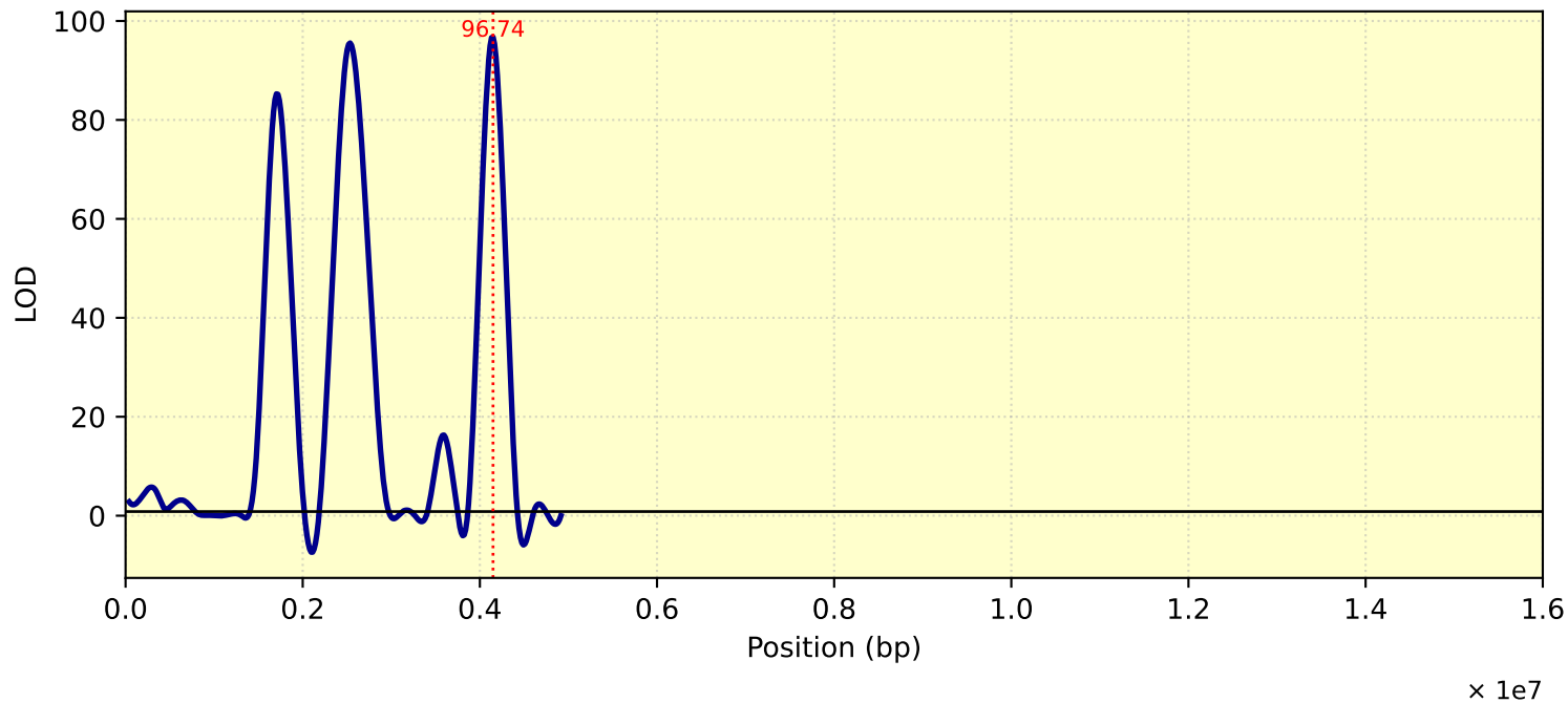
LOD Curve - chr12 - Tc30me2
