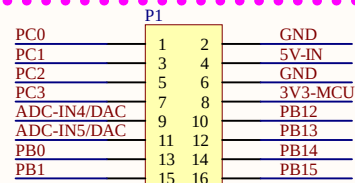
Header 8X2
