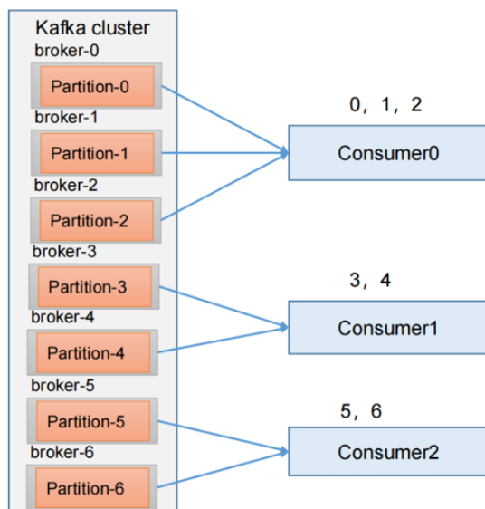
图 9: Range 策略
