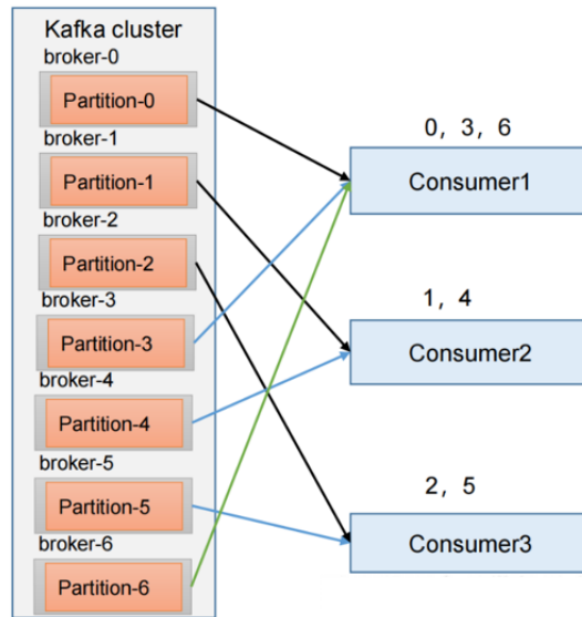
图 10: RoundRobin 策略
