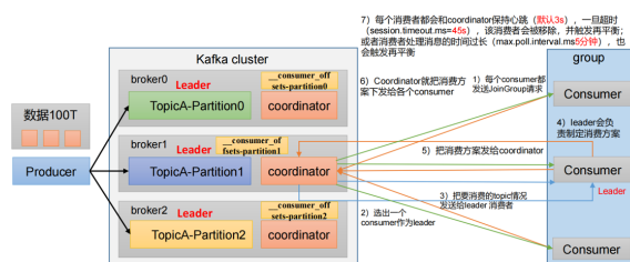
图 6: 消费者组的运行逻辑
