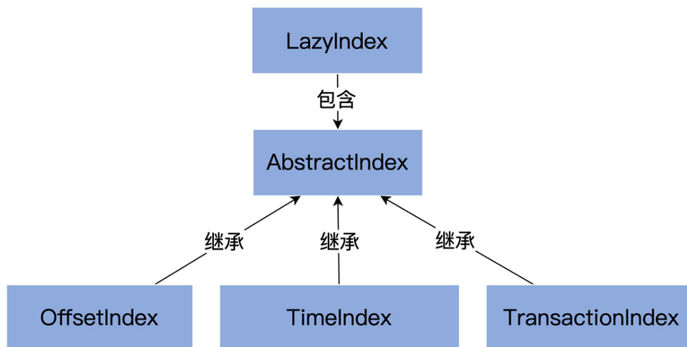
图 3: 五类索引之间的关系
