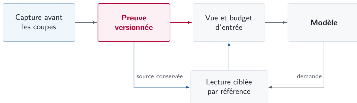
Figure 2 – Architecture proposée, non implémentée. La capture porte son statut de complétude ; la vue indique ses omissions. Une lecture ciblée récupère une source existante, sans rejouer l’action qui l’a produite.
