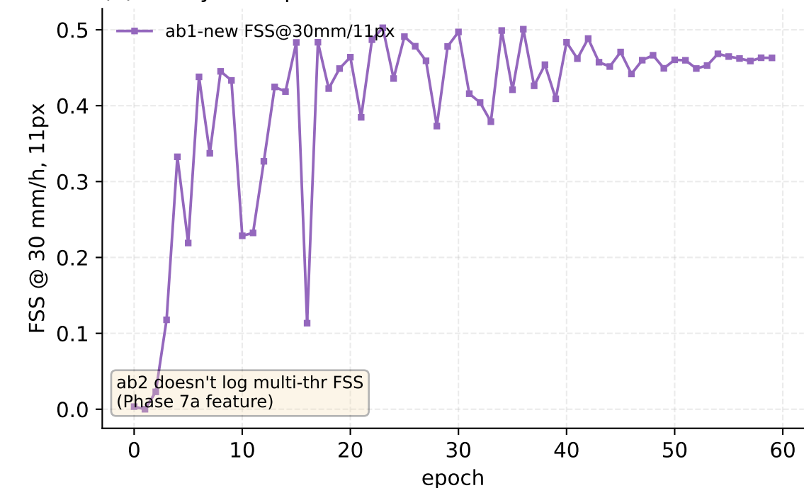
(d) Heavy-rain spatial skill
