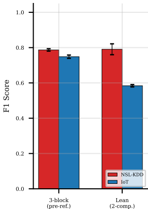
(a) F1
