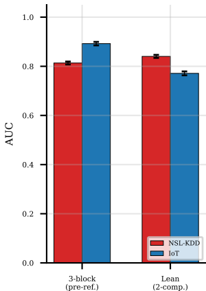
(b) AUC
