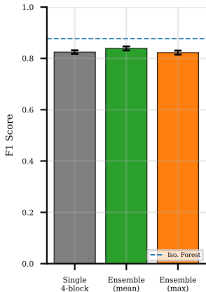
(b) Ensemble Effect on F1
