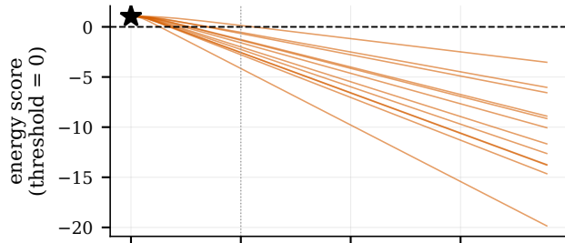
ViT-B/16
