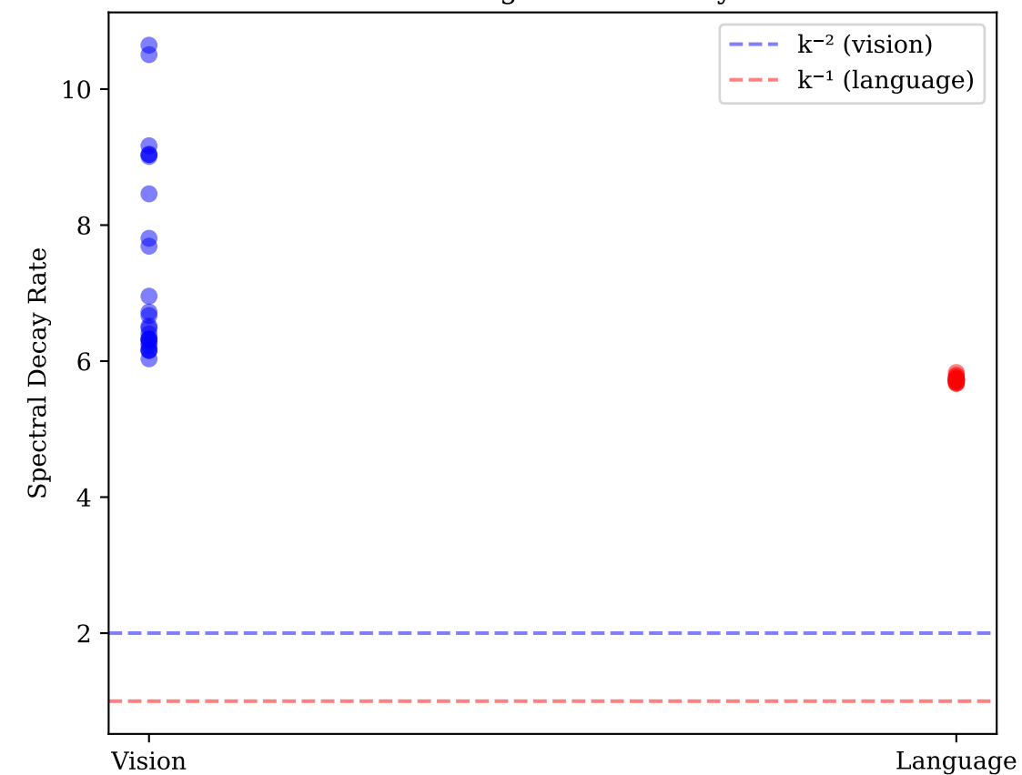
AGOP Eigenvalue Decay
