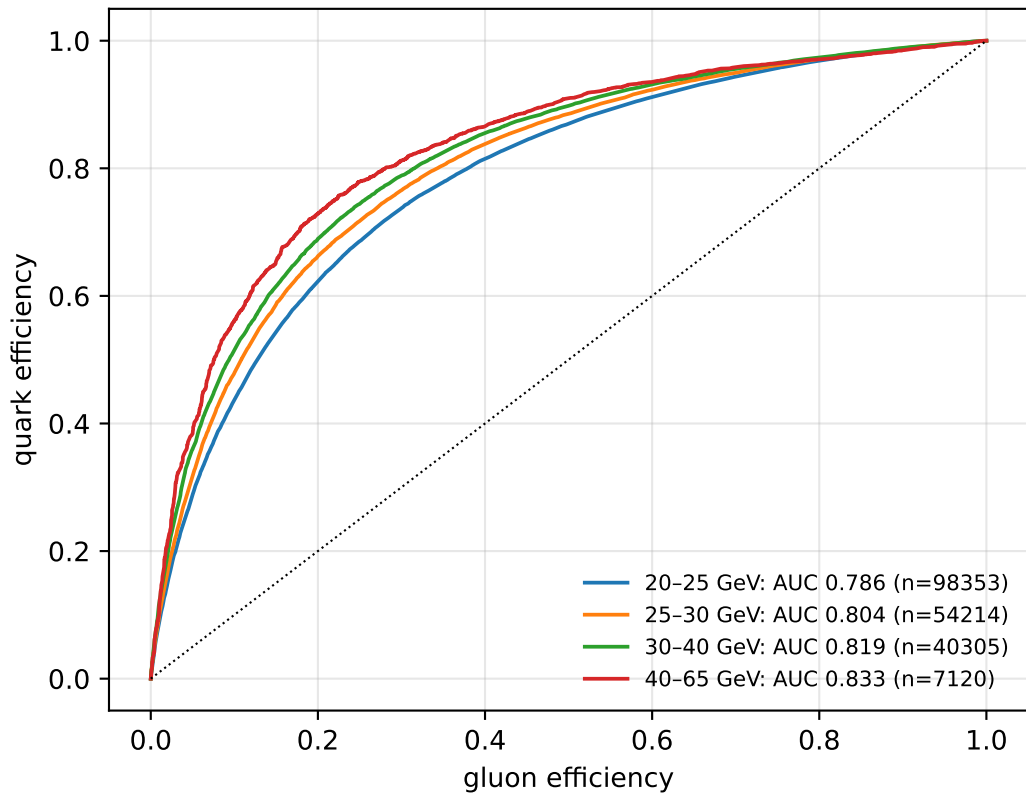
ROC per jet-pT bin
