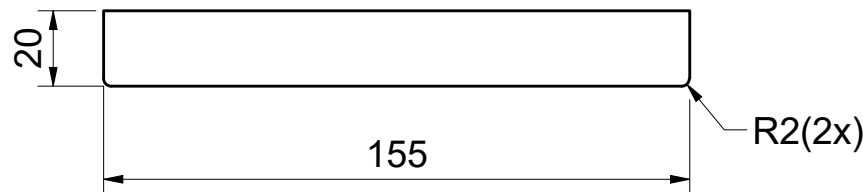
DETAIL-2 ( 1 : 2 )
