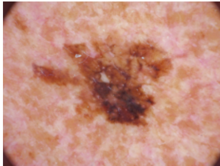
Maximum RGB
