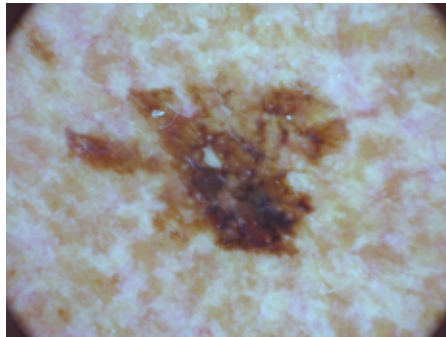
Gray World
