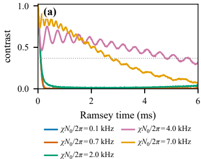
mean field, Voigt line
