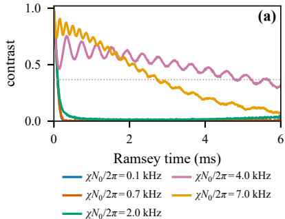
mean field, Voigt line
