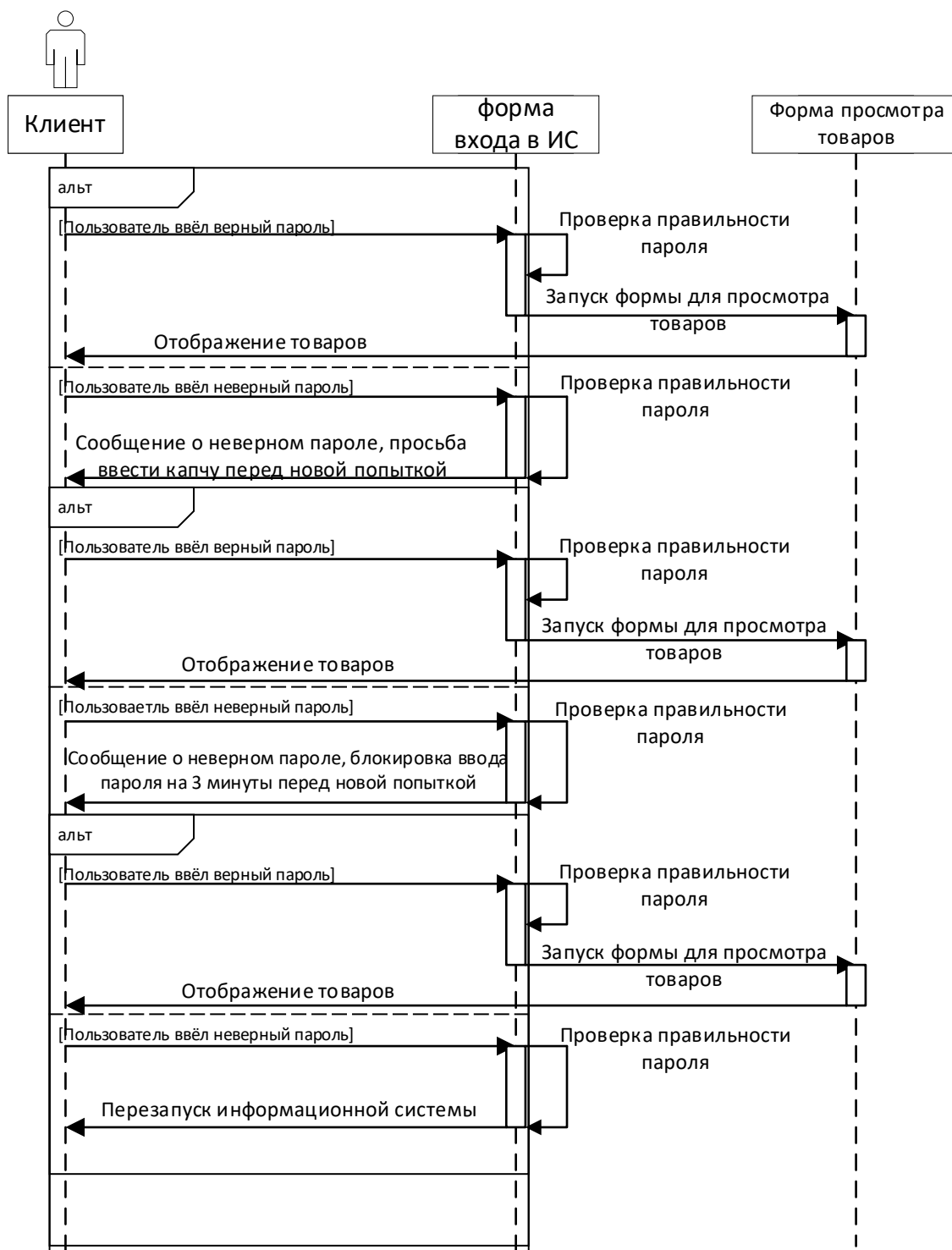
Рисунок 2 - Диаграмма последовательностей
