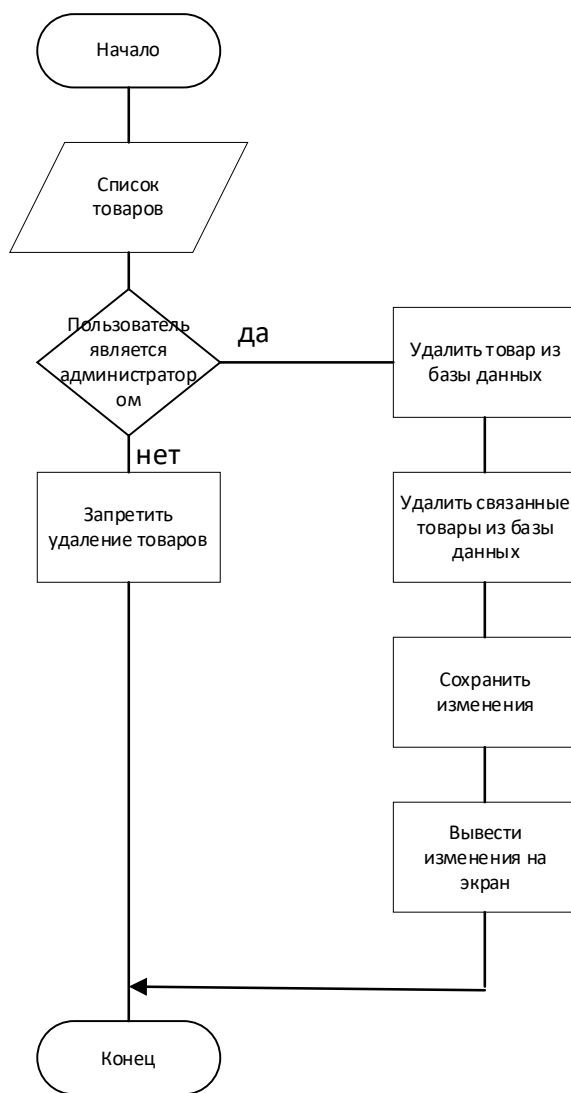
Рисунок 4 - Блок-схема функции удаления товаров
