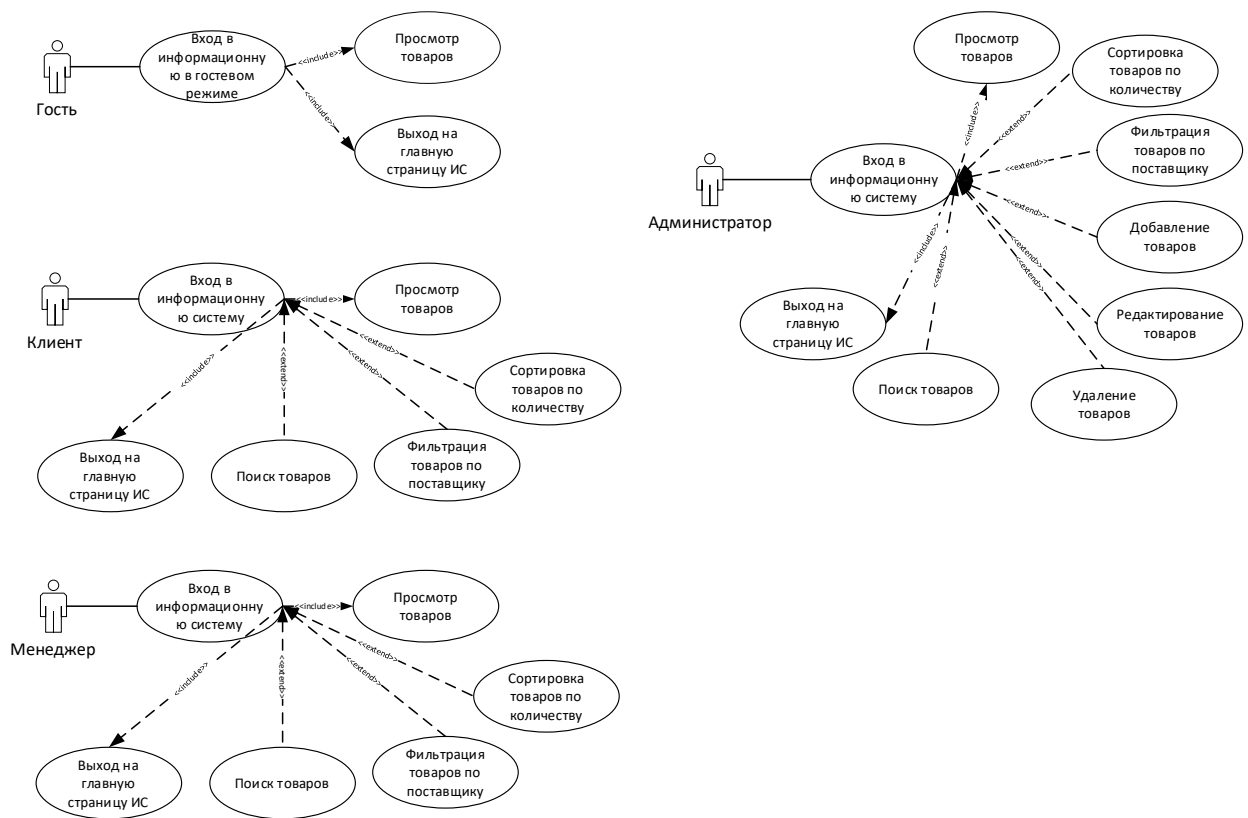
Рисунок 1 - Диаграмма претендентов
