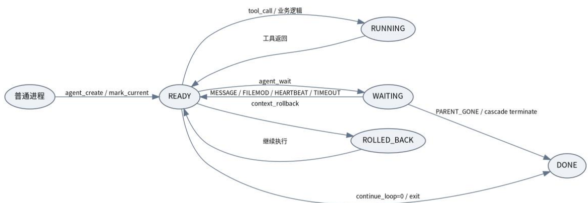
图 3.5 Loop 状态机
