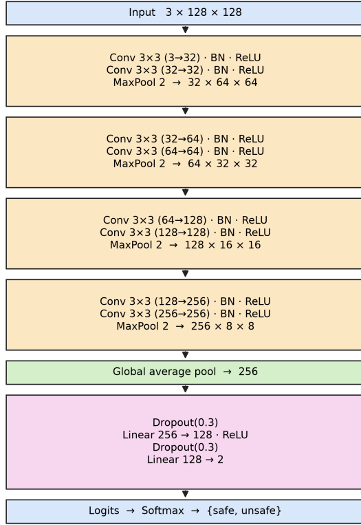
Scratch CNN — about 1.2M parameters
