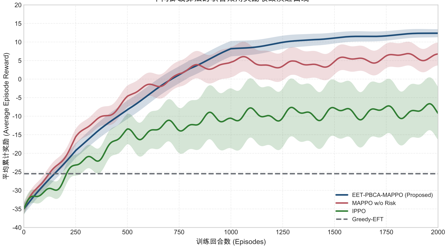
不同卸载算法的联合效用奖励收敛演进曲线
